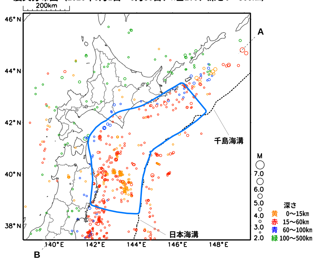
震央分布図 (2026年9月1日～9月30日、 M \geq 2.0 、深さ0～500km)
