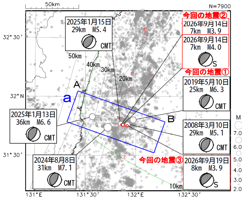
震央分布図 (1997年10月1日～2026年9月24日、深さ0～60km、 M \geq 2.0 ) 2026年9月14日以降の地震を赤色で表示
