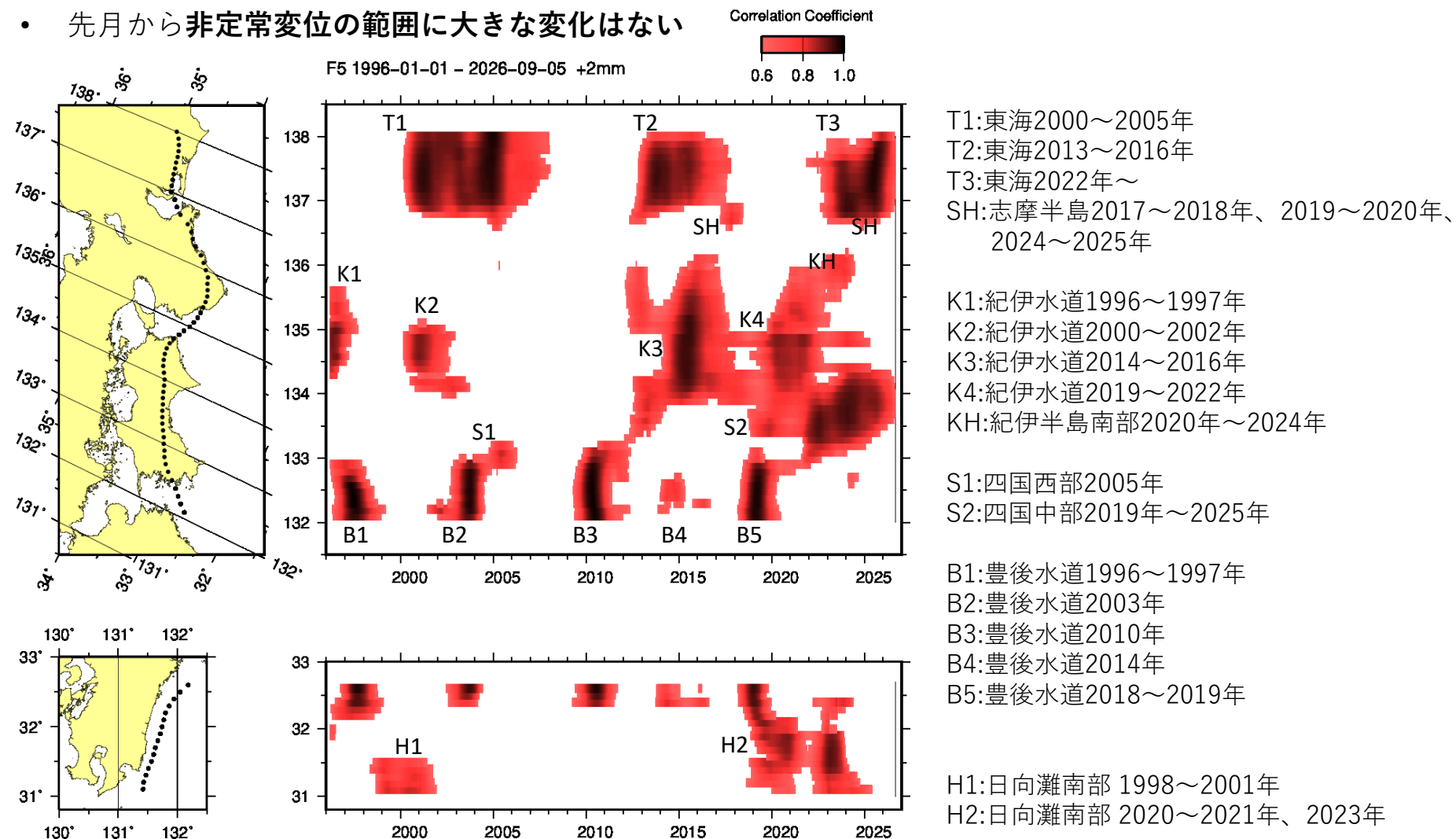
第1図 長期的スロースリップ客観検知図（1996年～2026年9月）
