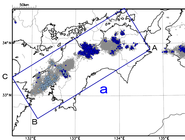
震央分布図 (2020年9月1日～2026年10月5日、 深さ0～60km、Mすべて)
