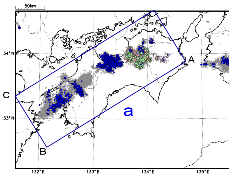
震央分布図 (2020年9月1日～2026年9月30日、 深さ0～60km、Mすべて)
