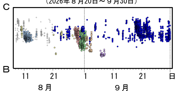
領域a内の時空間分布図 (B－C投影) (2026年8月20日～9月30日)
