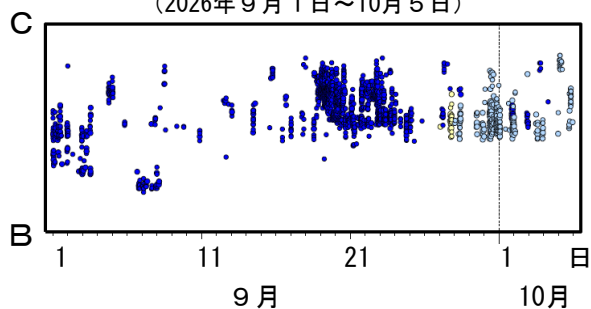
領域a内の時空間分布図 (B－C投影) (2026年9月1日～10月5日)
