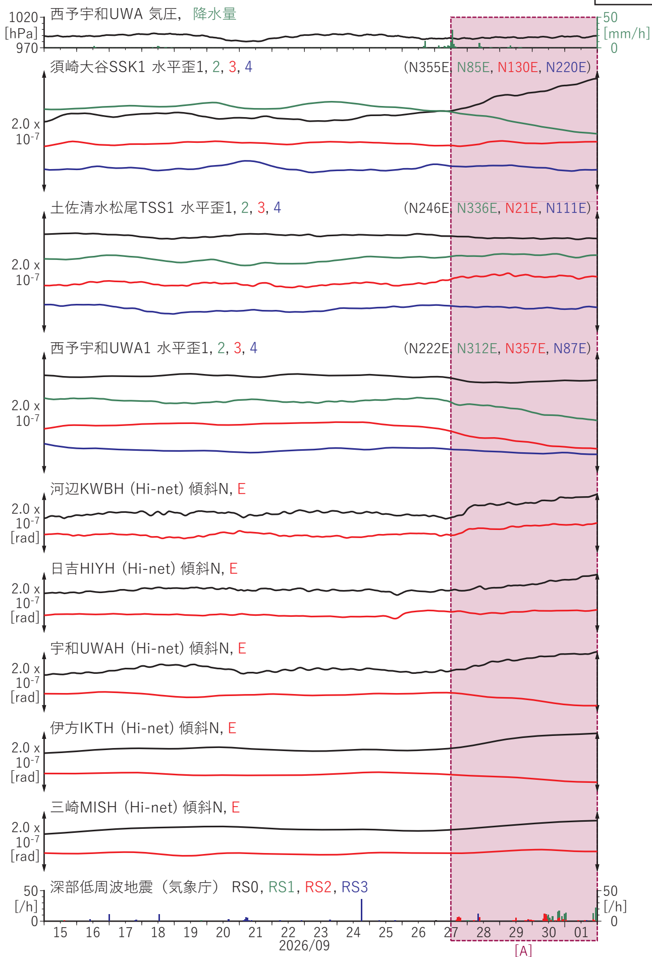
図11 四国地方における歪・傾斜観測結果 (2026/09/15 00:00 - 2026/10/02 00:00 (JST))
