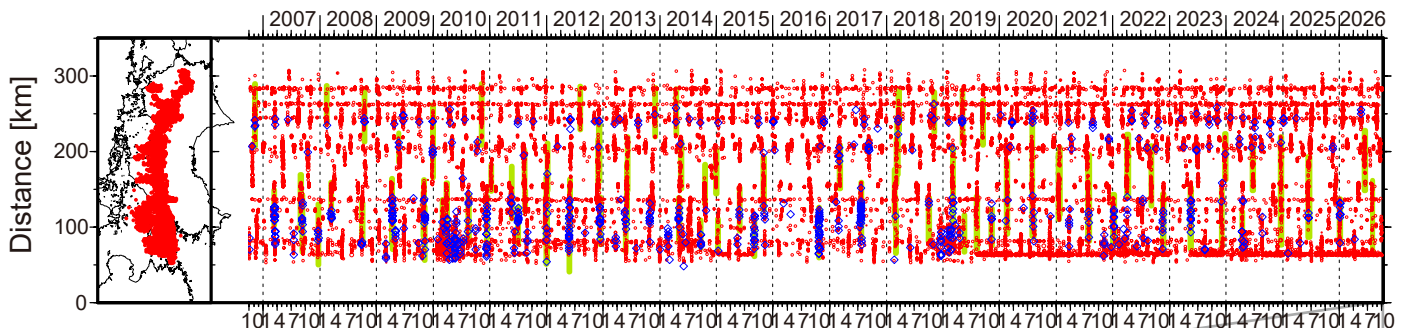
図 1. 四国における 2006 年 10 月～2026 年 10 月 4 日までの深部低周波微動の時空間分布 (上図). 赤丸はエンベロープ相関・振幅ハイブリッド法 (Maeda and Obara, 2009) およびクラスタ処理 (Obara et al., 2010) によって 1 時間毎に自動処理された微動分布の重心である. 青菱形は周期 20 秒に卓越する超低周波地震 (Ito et al., 2007) である. 黄緑色太線は、これまでに検出された短期的スロースリップイベント (SSE) を示す. 下図は 2026 年 9 月を中心とした期間の拡大図である. 8 月 27 日～9 月 7 日頃には、徳島県中部から愛媛県東部において、活発な微動活動がみられた. この活動は愛媛・香川・徳島県境付近で開始し、29 日頃から活発化するとともに東西両方向への拡大がみられた. 9 月 18～23 日頃には愛媛県東部において活発な活動がみられ、活動開始後から 20 日頃にかけてやや東方向に活動域が拡大したのち、21 日頃からは西側でも活動がみられた. 9 月 29 日～10 月 1 日頃には愛媛県西部において、小規模な活動がみられた. 10 月 1 日頃には香川県付近において、ごく小規模な活動がみられた.
