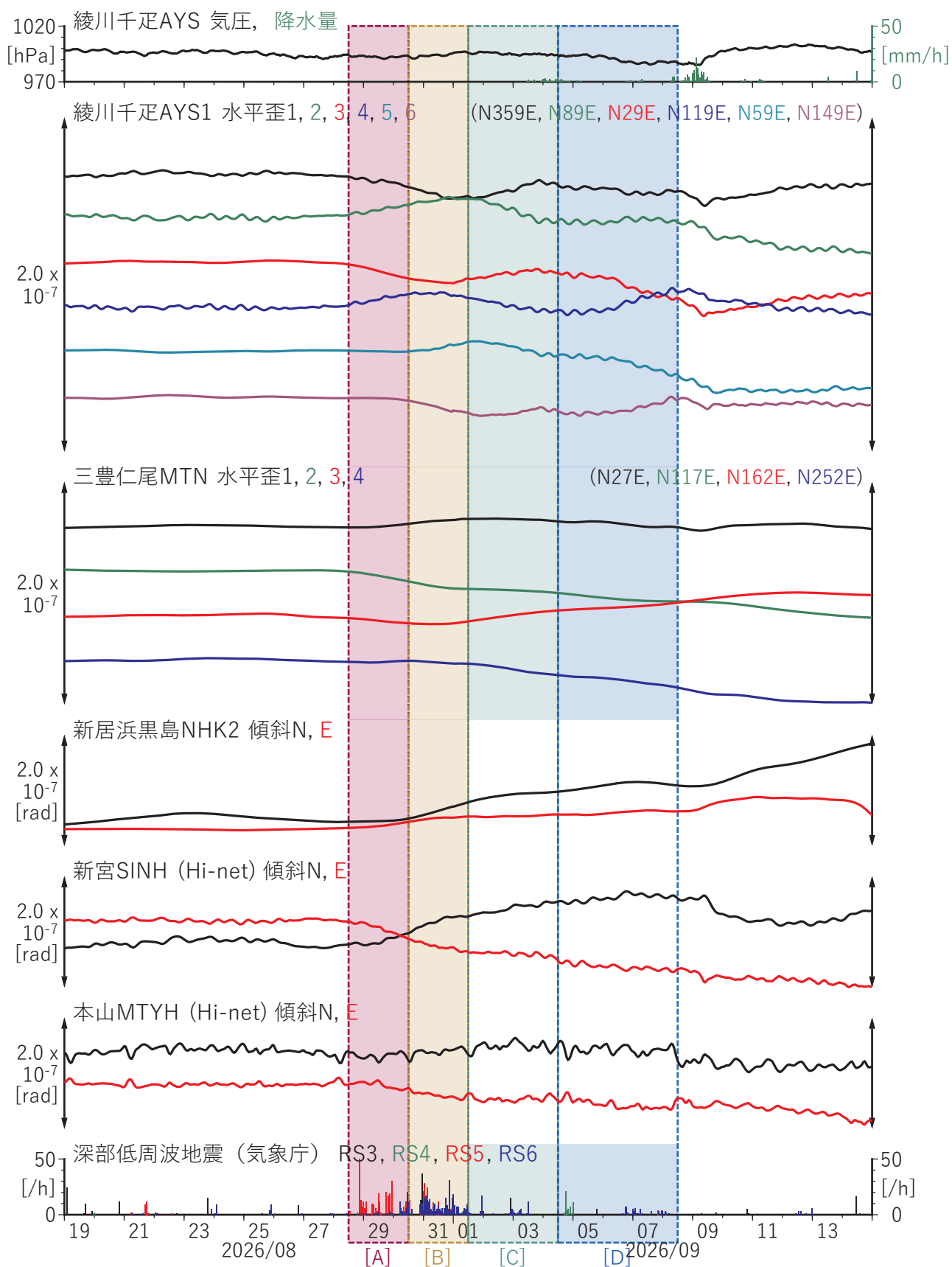
図2 四国地方における歪・傾斜観測結果 (2026/08/19 00:00 - 2026/09/15 00:00 (JST))
