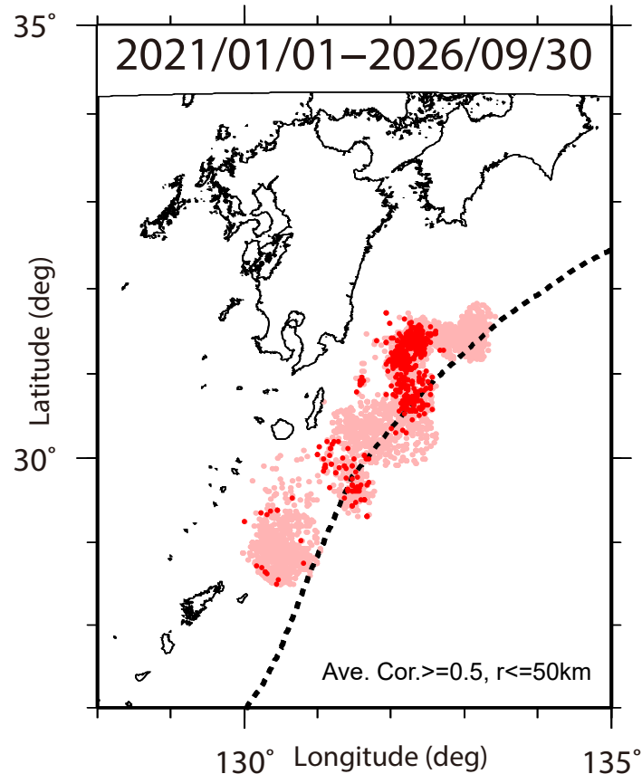
第1図. 2021年1月1日から2026年9月30日までの期間内に波形相関解析 [Asano et al. (2015)] によって検出された超低周波イベントの震央分布. 検出イベントを防災科研の手動または自動検測震源と照合して通常の地震を除去した後に, それ以外を超低周波イベントとして桃色 (2026年6月30日以前), および赤色 (2026年7月1日以降) の点でそれぞれ示す.
