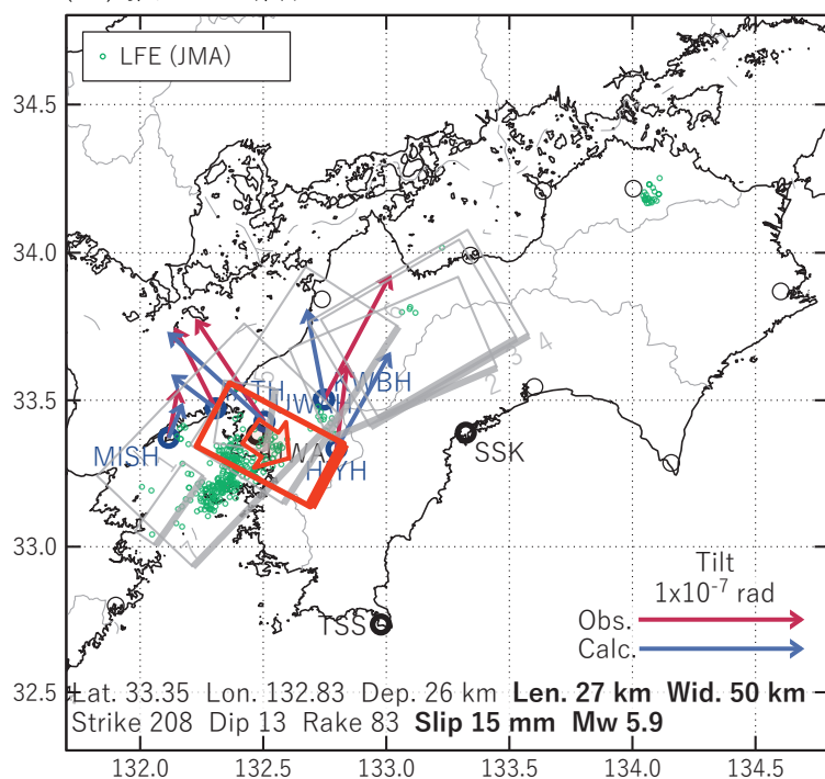
図12 2026/09/27PM-10/01の歪・傾斜変化(図11[A])を説明する断層モデル。
