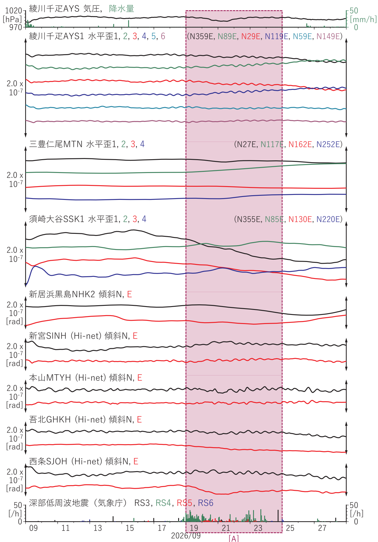
図8 四国地方における歪・傾斜観測結果 (2026/09/09 00:00 - 2026/09/29 00:00 (JST))
