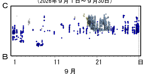
領域a内の時空間分布図（B－C投影） (2026年9月1日～9月30日)
