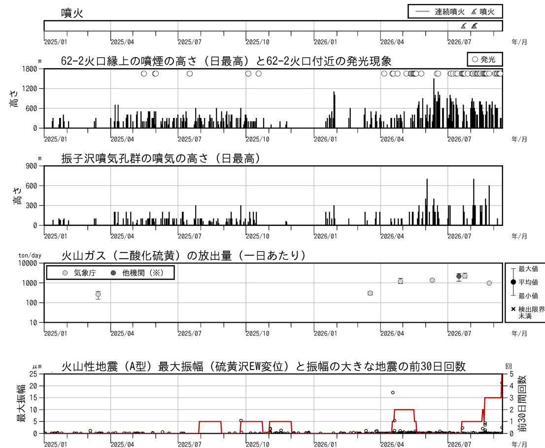
図 十勝岳 火山活動経過図(2025年1月1日 ～ 2026年9月12日)
