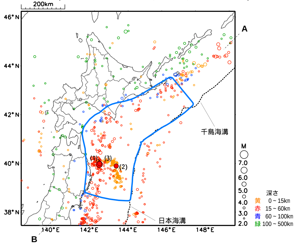
震央分布図（2026年7月1日～7月31日、M 2.0、深さ0～500km）
