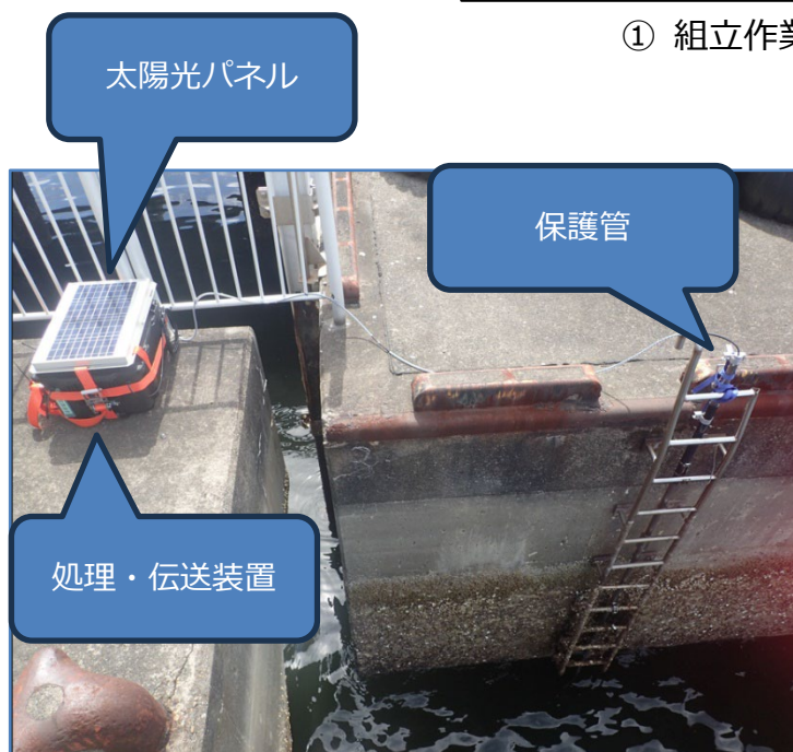
② 装置全体図
