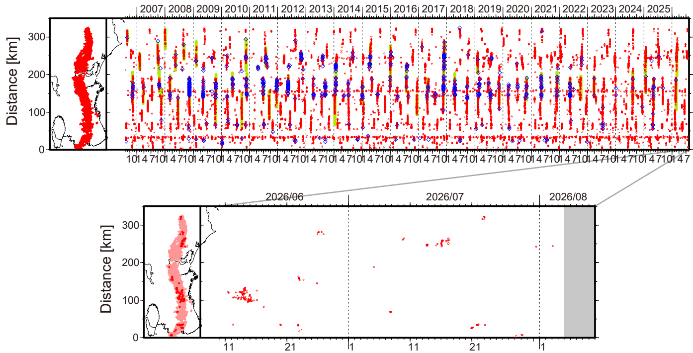
図 1. 紀伊半島・東海地域における 2006 年 8 月～2026 年 8 月 4 日までの深部低周波微動の時空間分布(上图)．赤丸はエンベロープ相関・振幅ハイブリッド法 (Maeda and Obara, 2009) およびクラスタ処理 (Obara et al., 2010) によって 1 時間毎に自動処理された微動分布の重心である．青菱形は周期 20 秒に卓越する超低周波地震(Ito et al., 2007)である．黄緑色の太線はこれまでに検出された短期的スロースリップイベント(SSE)を示す．下图は 2026 年 7 月を中心とした期間の拡大図である．7 月以降の期間について顕著な活動はとくにみられなかったものの、7 月 13 日頃には愛知県中部でごく小規模な活動がみられた．その後 7 月 15～17 日頃には愛知県中部から東部で小規模な活動がみられ、13 日の活動域付近から東方向への活動域の拡大がみられた．7 月 20～23 日頃には、和歌山県中部において小規模な活動がみられ、7 月 28～29 日頃には同活動域の西側でごく小規模な活動がみられた．
