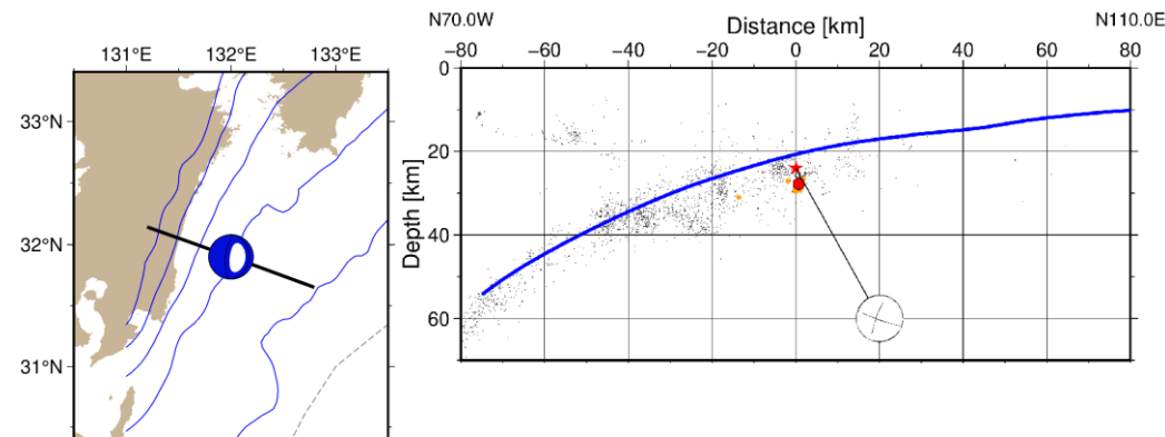
図2 鉛直断面におけるプレート上面モデル(青線:Nakanishi et al., 2018)との対比. 赤星はセントロイド位置を表す. Nakanishi et al. (2025)による三次元地震波速度構造を用いて求めた M \geq 1.0 の地震の震源位置(黒:2003/01/01-2026/08/02, 橙:2026/08/02-2026/08/04)及び M \geq 5.5 の地震の震源位置(赤丸:2026/08/02-2026/08/04)を背景に示す..ただし、鉛直断面図には最適ダブルカップル解の節面のみを示す.
