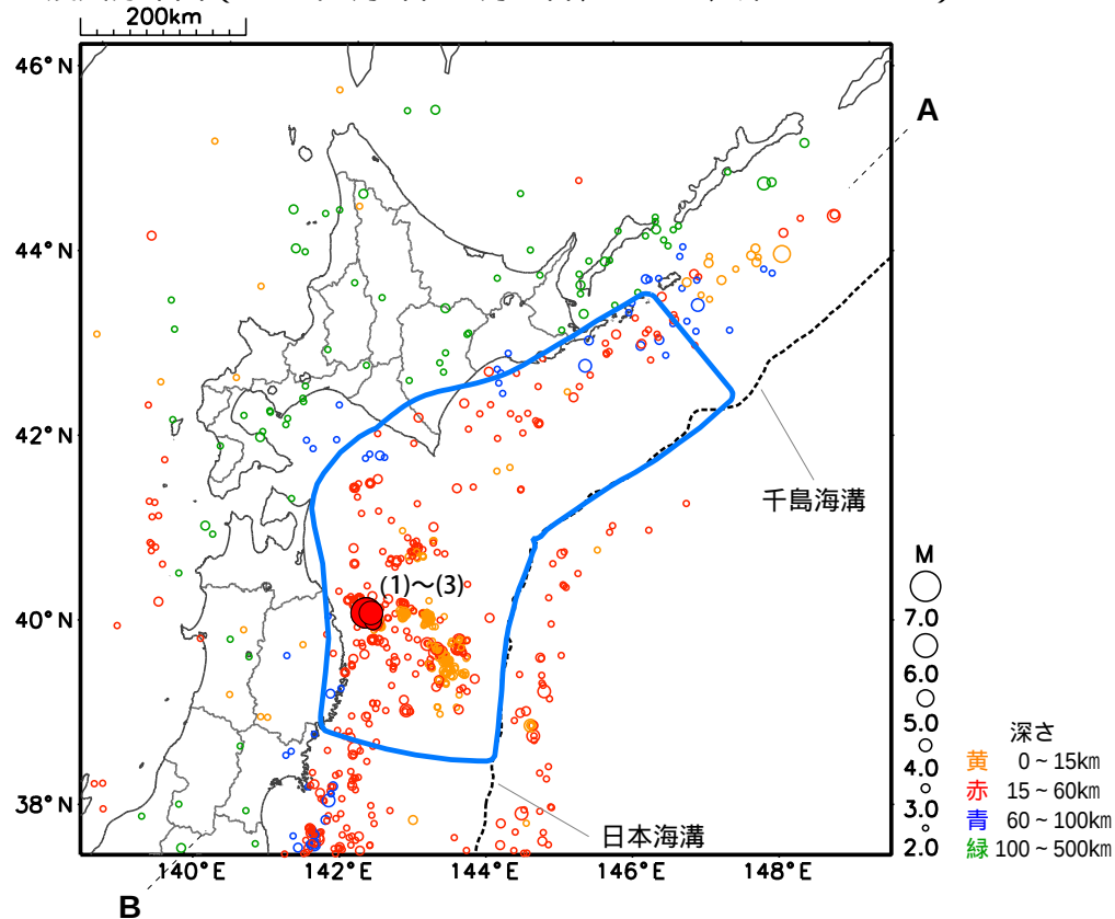
震央分布図（2026年6月1日～6月30日、M 2.0、深さ0～500km）
