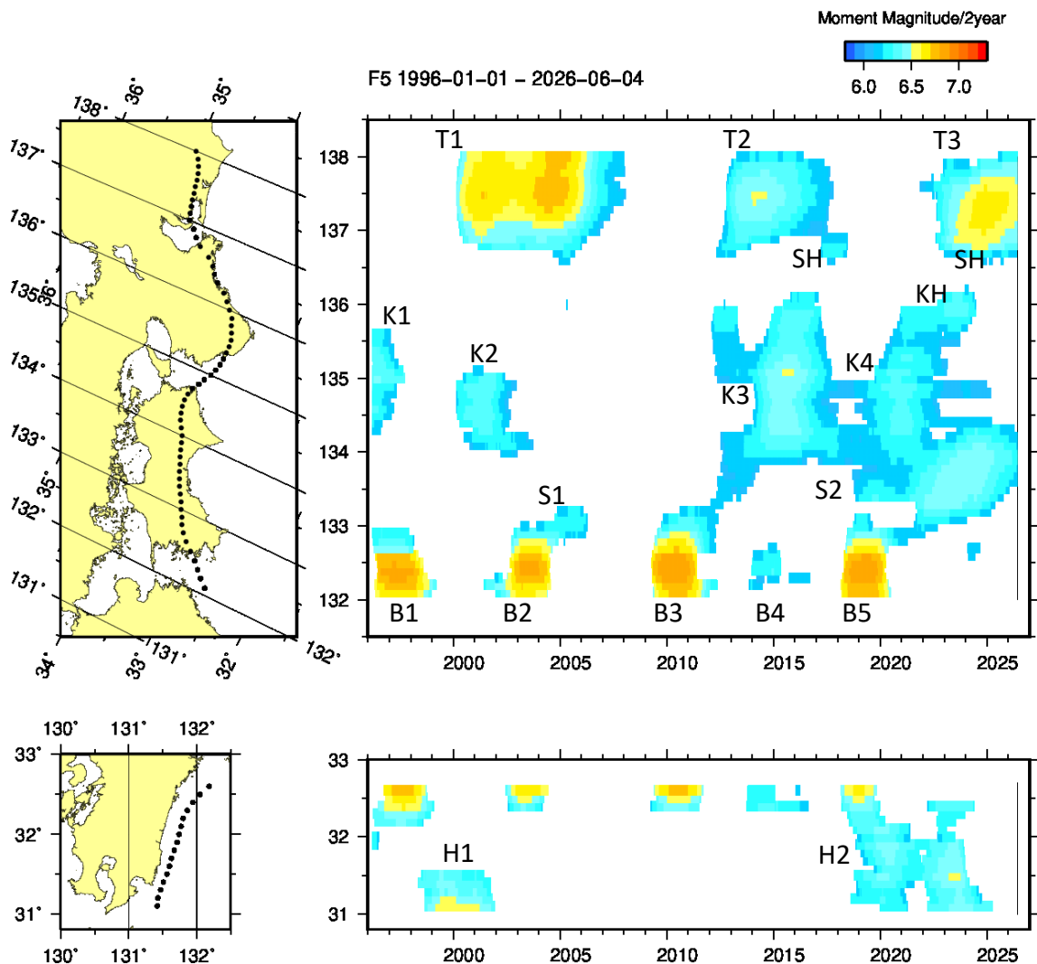
第2図 長期的スロースリップの規模分布 (1996年～2026年6月) 2年間あたりの変化量から推定したモーメントマグニチュード。
