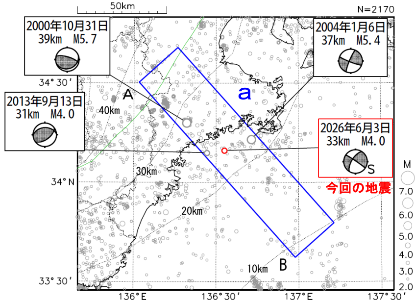
震央分布図 (1997年10月1日~2026年6月3日、深さ0~80km、M≥2.0) 2026年6月3日の地震を赤色で表示
