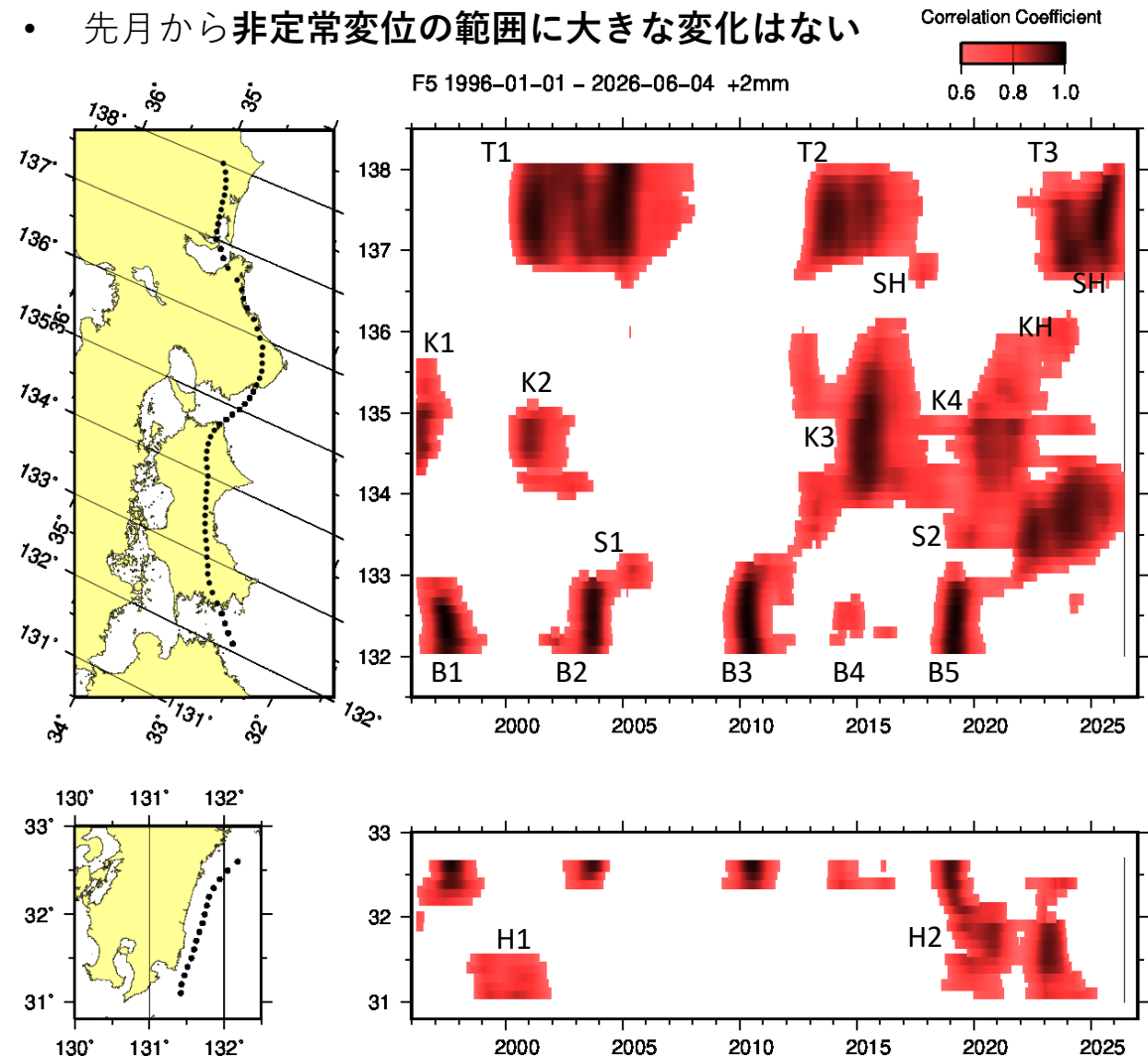
第1図 長期的スロースリップ客観検知図（1996年～2026年6月）
