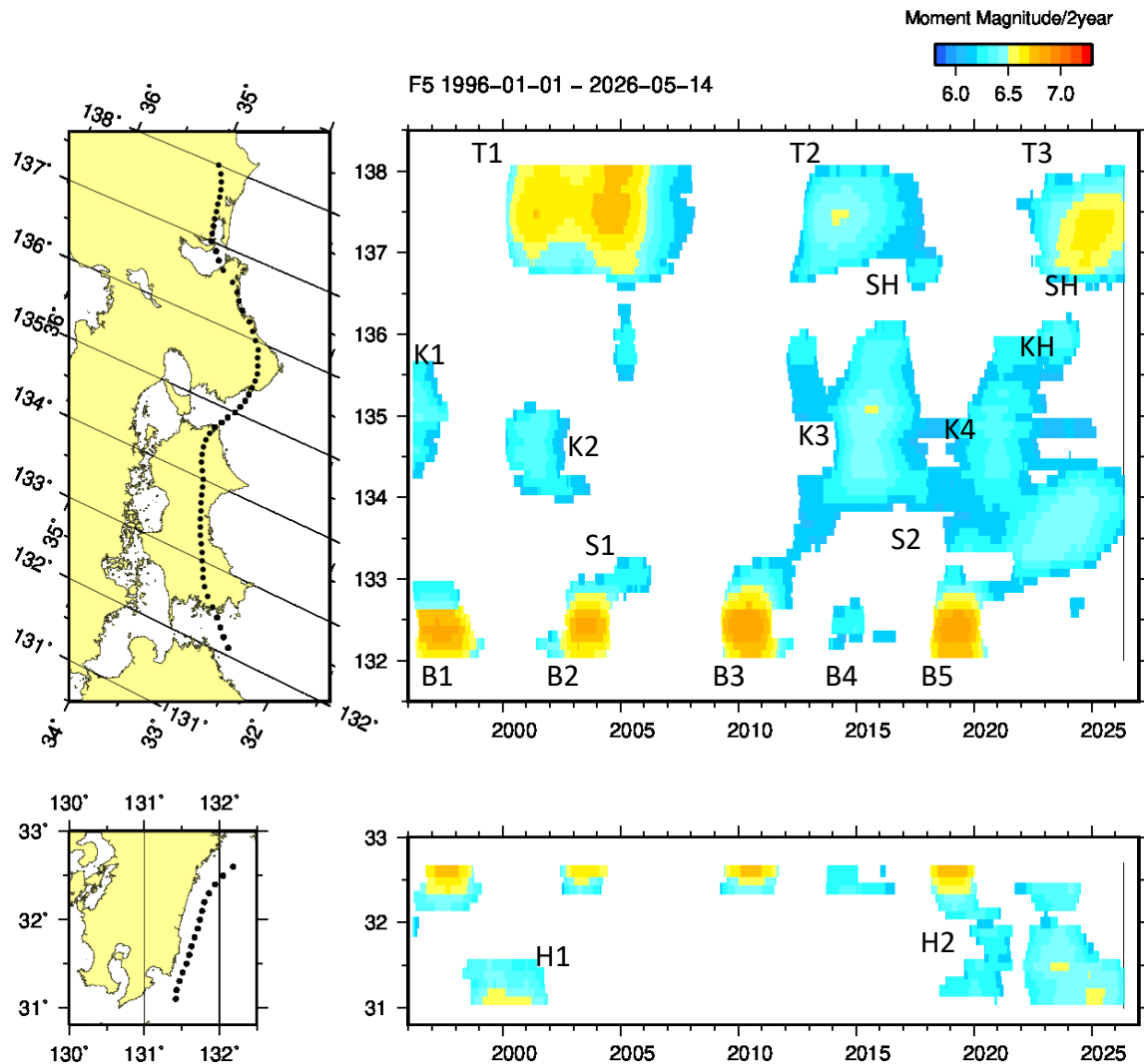
第2図 長期的スロースリップの規模分布 (1996年～2026年5月) 2年間あたりの変化量から推定したモーメントマグニチュード。
