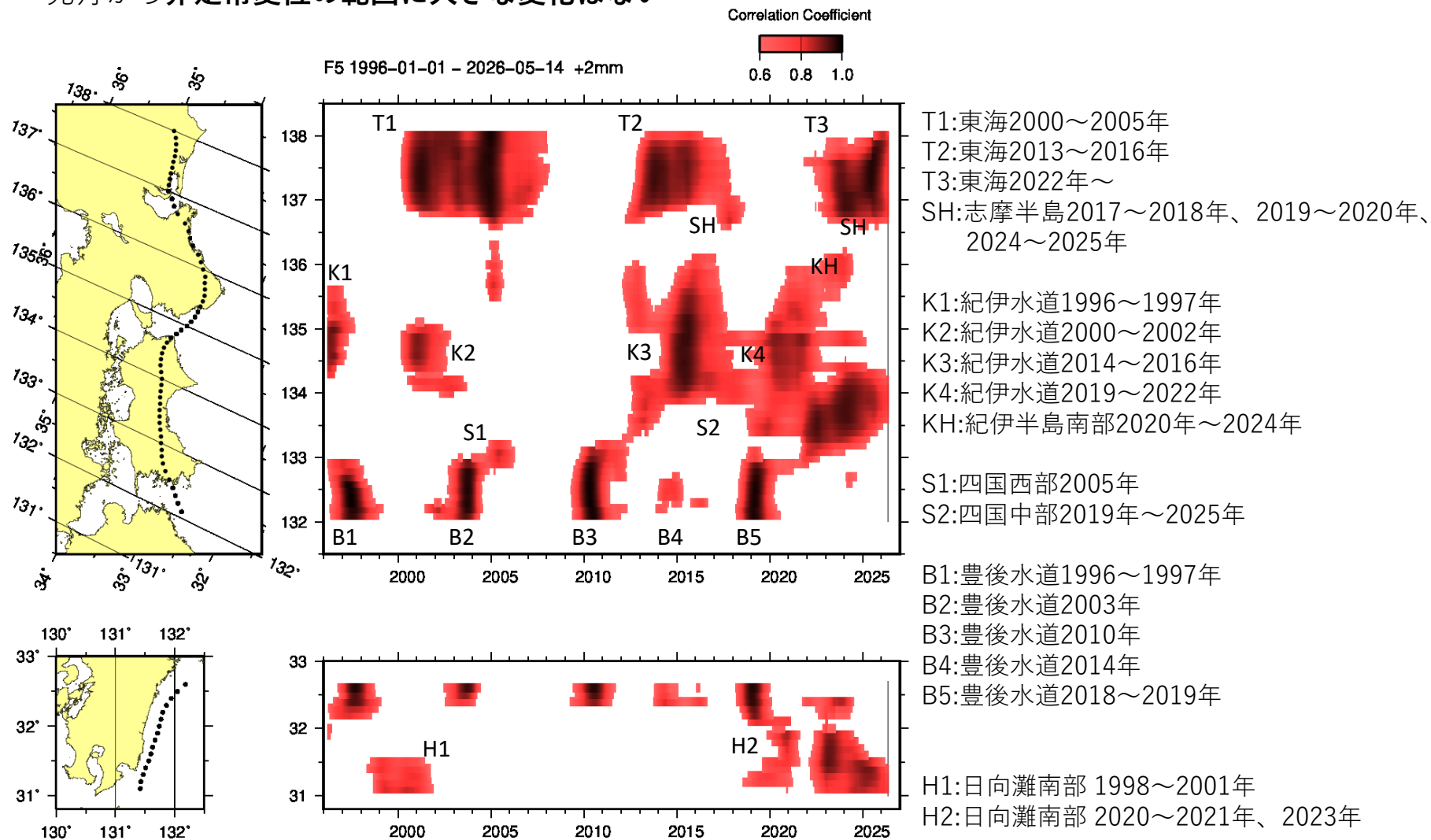
第1図 長期的スロースリップ客観検知図（1996年～2026年5月）
