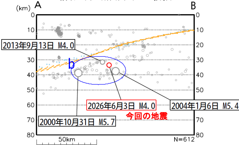
領域 a 内の断面図 (A-B 投影)
