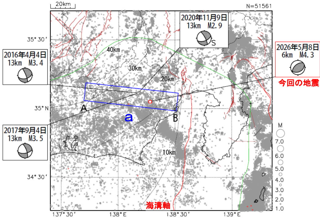
震央分布図 (1997年10月1日～2026年5月9日、深さ0～60km、M≥1.0) 2026年5月8日以降の地震を赤色で表示
