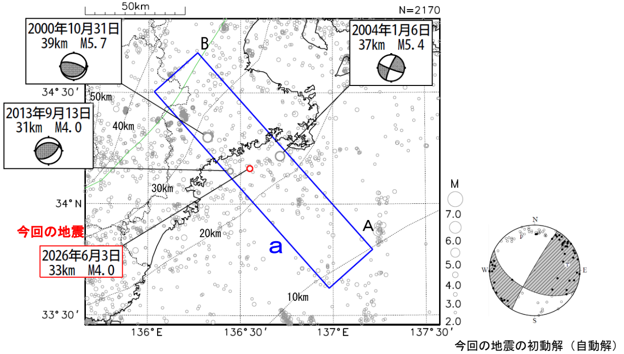
震央分布図 (1997年10月1日～2026年6月3日、深さ0～80km、 M \geq 2.0 ) 2026年6月3日の地震を赤色、 それ以外の期間の地震を灰色で表示
