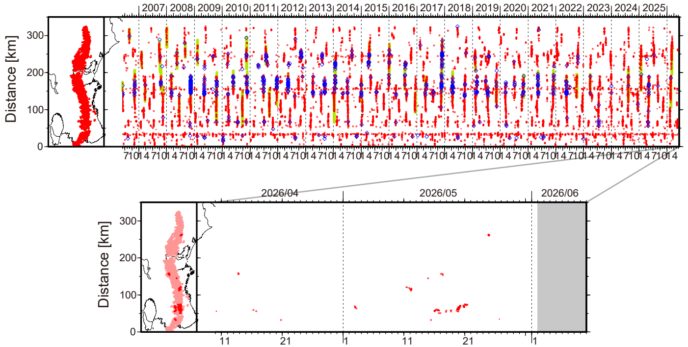
図1. 紀伊半島・東海地域における2006年6月～2026年6月1日までの深部低周波微動の時空間分布(上図). 赤丸はエンベロープ相関・振幅ハイブリッド法 (Maeda and Obara, 2009) およびクラスタ処理 (Obara et al., 2010) によって1時間毎に自動処理された微動分布の重心である. 青菱形は周期20秒に卓越する超低周波地震 (Ito et al., 2007) である. 黄緑色の太線はこれまでに検出された短期的スロースリップイベント (SSE) を示す. 下図は2026年5月を中心とした期間の拡大図である. 5月16～21日頃には奈良県南部でやや活発な微動活動がみられた. この活動は、奈良・和歌山県境付近で開始し、やや北東方向への活動域の移動がみられた. 5月2～3日頃には奈良県南部において、5月11～12日頃には三重県南部において、5月24～25日頃には愛知県東部において、それぞれごく小規模な活動がみられた.
