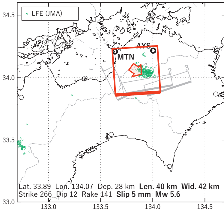
図9 2026/05/09PM-15AMの歪変化 (図8[A]) を説明する断層モデル。
