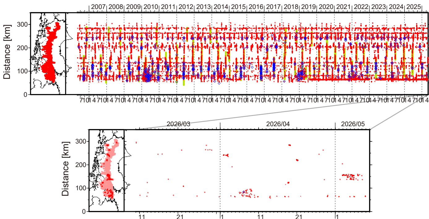
図1. 四国における2006年5月～2026年5月9日までの深部低周波微動の時空間分布(上図). 赤丸はエンベロープ相関・振幅ハイブリッド法 (Maeda and Obara, 2009) およびクラスタ処理 (Obara et al., 2010) によって1時間毎に自動処理された微動分布の重心である. 青菱形は周期20秒に卓越する超低周波地震 (Ito et al., 2007) である. 黄緑色太線は、これまでに検出された短期的スロースリップイベント (SSE) を示す. 下図は2026年4月を中心とした期間の拡大図である. 4月6～10日頃には豊後水道付近において、やや活発な活動がみられた. この活動は沈み込むプレートの深部側から開始し、浅部側への活動域の拡大がみられた. 5月2～8日頃には愛媛県西部において活発な活動がみられ、やや西方向への活動域の拡大がみられた. 4月1～3日頃には愛媛・香川・徳島県境付近において小規模な微動活動がみられた. 4月18日頃には愛媛県西部において、4月18～19日頃には香川県付近において、4月20～21日頃には愛媛県東部において、それぞれごく小規模な活動がみられた.
