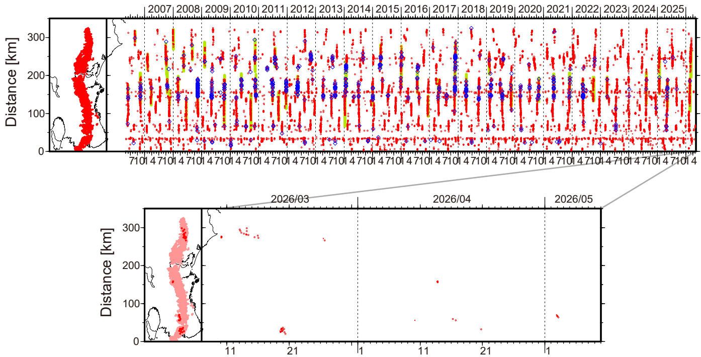
図1. 紀伊半島・東海地域における2006年5月～2026年5月9日までの深部低周波微動の時空間分布（上図）。赤丸はエンベロープ相関・振幅ハイブリッド法 (Maeda and Obara, 2009) およびクラスタ処理 (Obara et al., 2010) によって1時間毎に自動処理された微動分布の重心である。青菱形は周期20秒に卓越する超低周波地震 (Ito et al., 2007) である。黄緑色の太線はこれまでに検出された短期的スロースリップイベント (SSE) を示す。下図は2026年4月を中心とした期間の拡大図である。4月以降の期間について顕著な活動はみられなかったものの、4月13日頃には三重県北部において、5月2～3日頃には奈良県南部において、それぞれごく小規模な活動がみられた。
