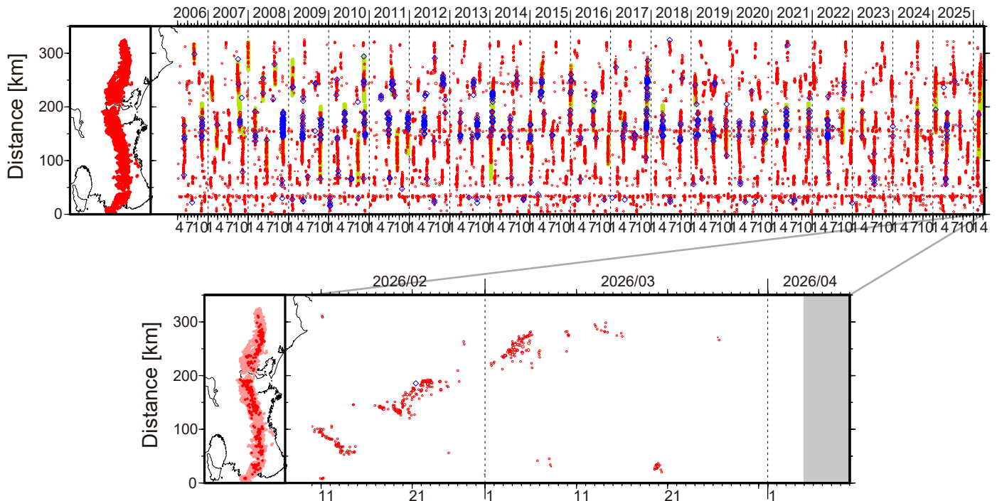
図1. 紀伊半島・東海地域における2006年4月～2026年4月4日までの深部低周波微動の時空間分布(上図). 赤丸はエンベロップ相関・振幅ハイブリッド法(Maeda and Obara, 2009)およびクラスタ処理(Obara et al., 2010)によって1時間毎に自動処理された微動分布の重心である. 青菱形は周期20秒に卓越する超低周波地震(Ito et al., 2007)である. 黄緑色の太線はこれまでに検出された短期的スロースリップイベント(SSE)を示す. 下図は2026年3月を中心とした期間の拡大図である. 3月1～7日頃に愛知県西部から愛知・長野県境付近において、活発な活動がみられた. この活動は愛知県西部から開始し、東方向への活動域の拡大がみられた. この活動に際し、傾斜変動から短期的SSEの断層モデルも推定されている. その後愛知・長野県境付近において、3月9～10日頃および3月13～16日頃に、それぞれごく小規模および小規模な活動がみられた. 後者の活動ではやや南西方向への活動域の移動がみられた. 和歌山県中部では、3月8日頃および3月19～20日頃に、それぞれごく小規模な活動がみられた.
