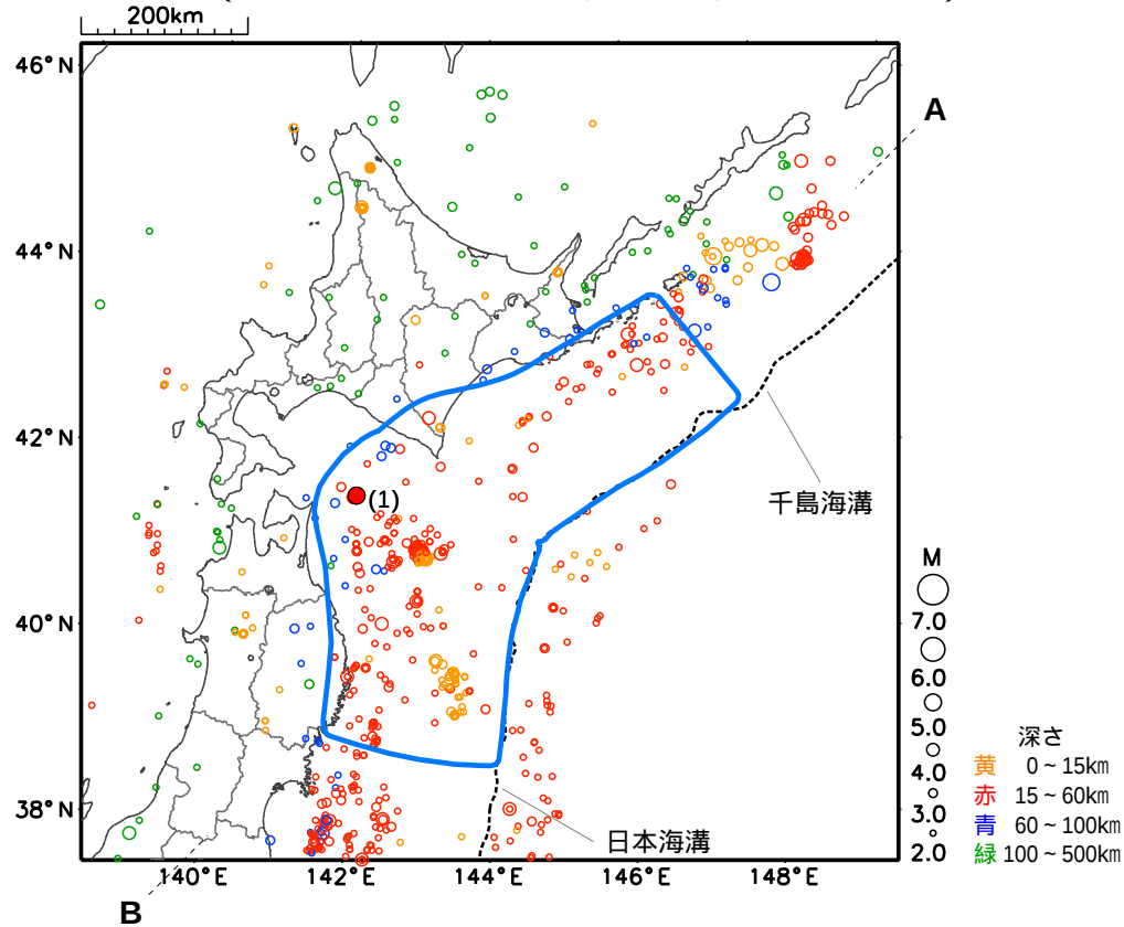
震央分布図（2026年2月1日～2月28日、M 2.0、深さ0～500km）
