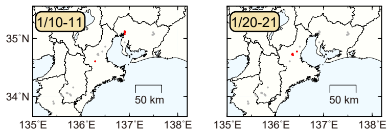
図 2. 各期間に発生した微動 (赤丸). 灰丸は, 図 1 の拡大図で示した期間における微動分布を示す.
