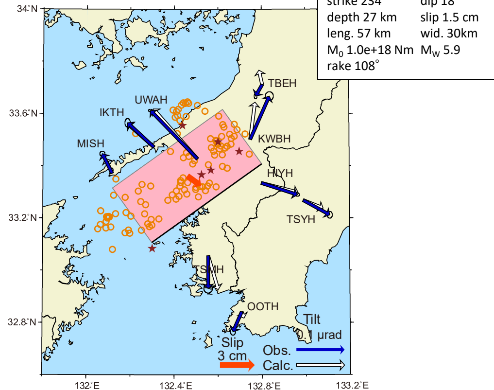
図2：1月1日～7日に観測された傾斜変化ベクトル（青矢印），推定されたスロースリップイベントの断層モデル（赤矩形・矢印），モデルから計算される傾斜変化ベクトル（白抜き矢印）を示す。1時間毎の微動エネルギーの重心位置（橙丸），深部超低周波地震（茶星印）も合わせて示す。すべり角はプレート相対運動方向に固定している。
