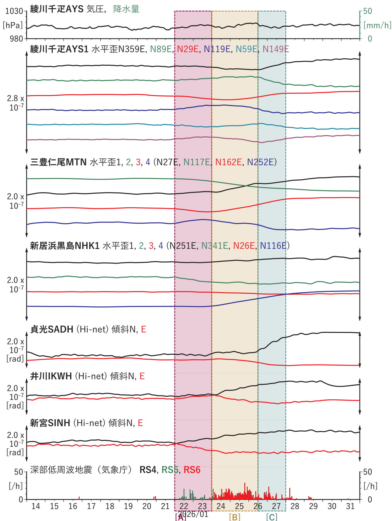
図9 歪・傾斜の時間変化 (2026/01/14 00:00–2026/02/01 00:00 (JST))
