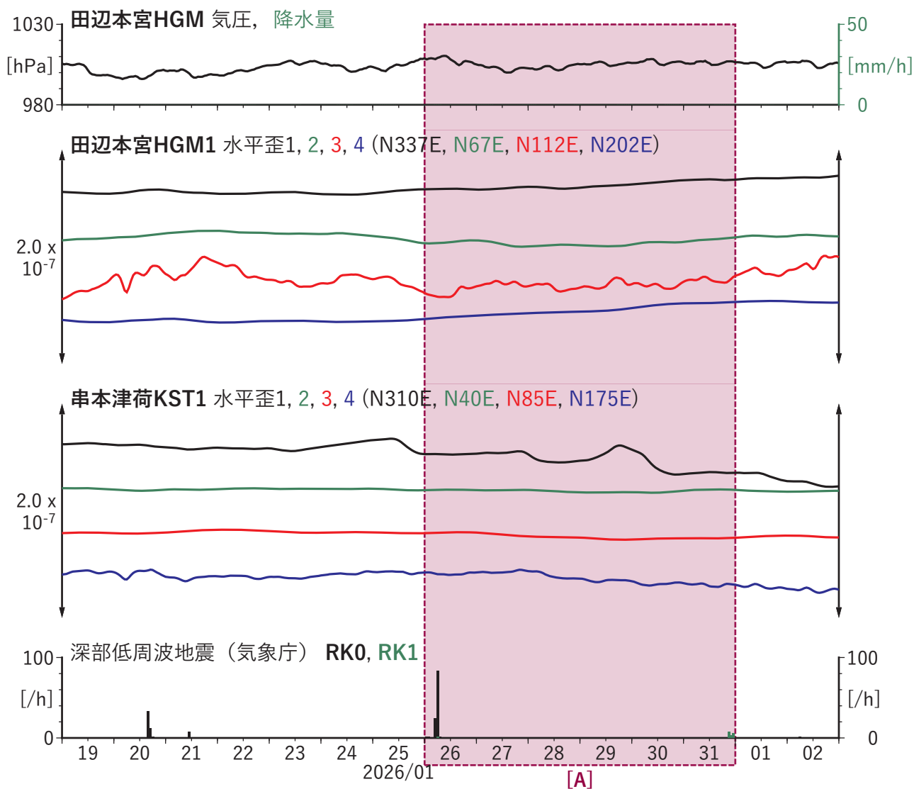
図2 歪の時間変化（2026/01/19 00:00–2026/02/03 00:00 (JST)）
