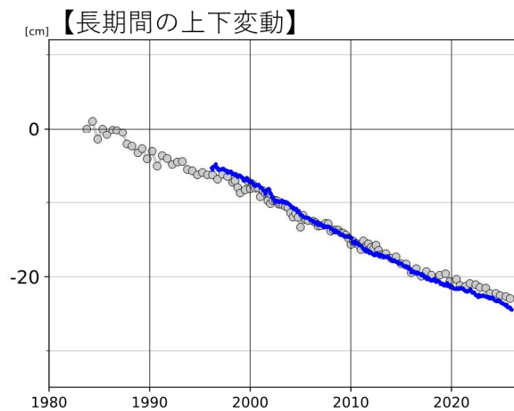
「固定局：掛川 A (161216)」
