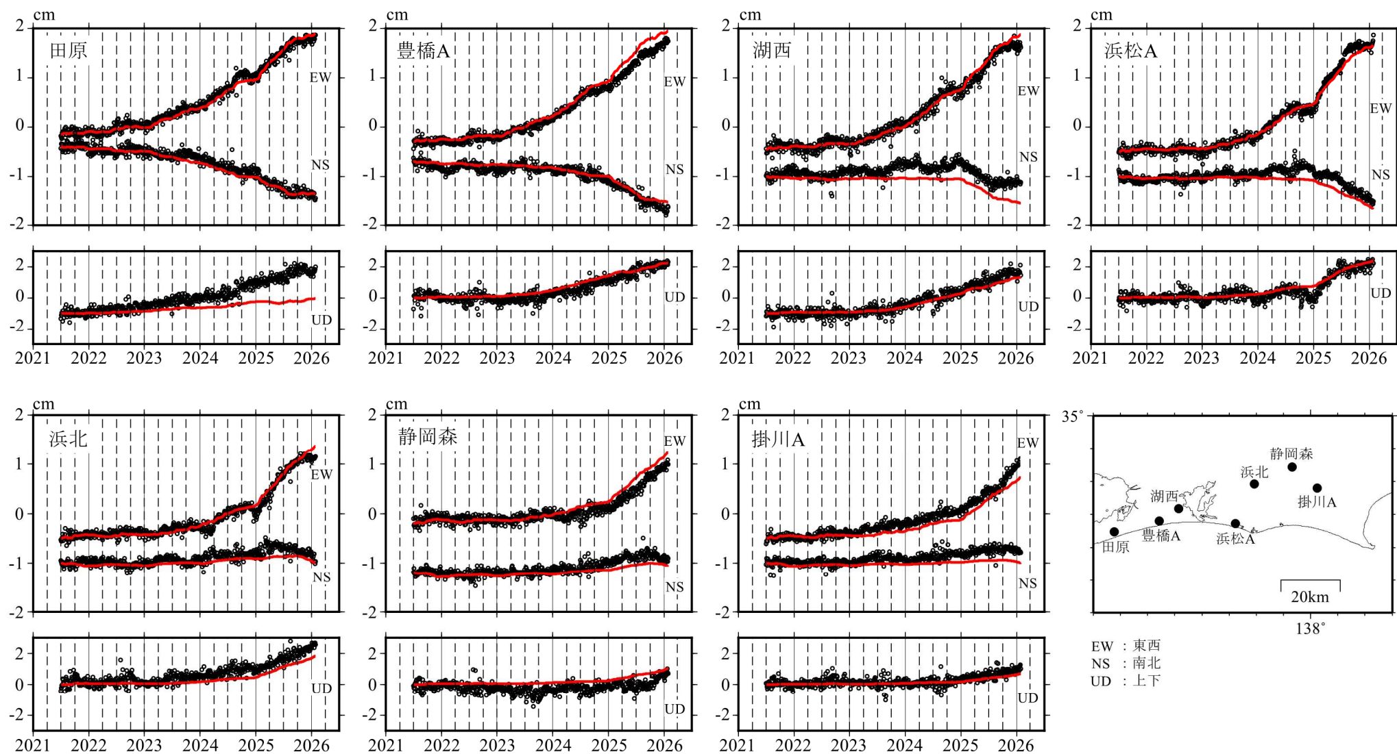
東海地域の観測点の座標時系列(黒丸)と計算値(赤線) 時間依存のインバージョン
