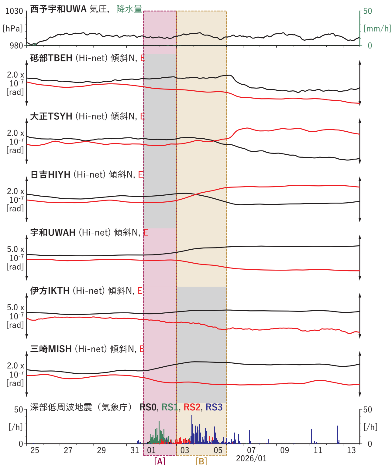
図5 歪・傾斜の時間変化(2) (2025/12/25 00:00–2026/01/14 00:00 (JST))
