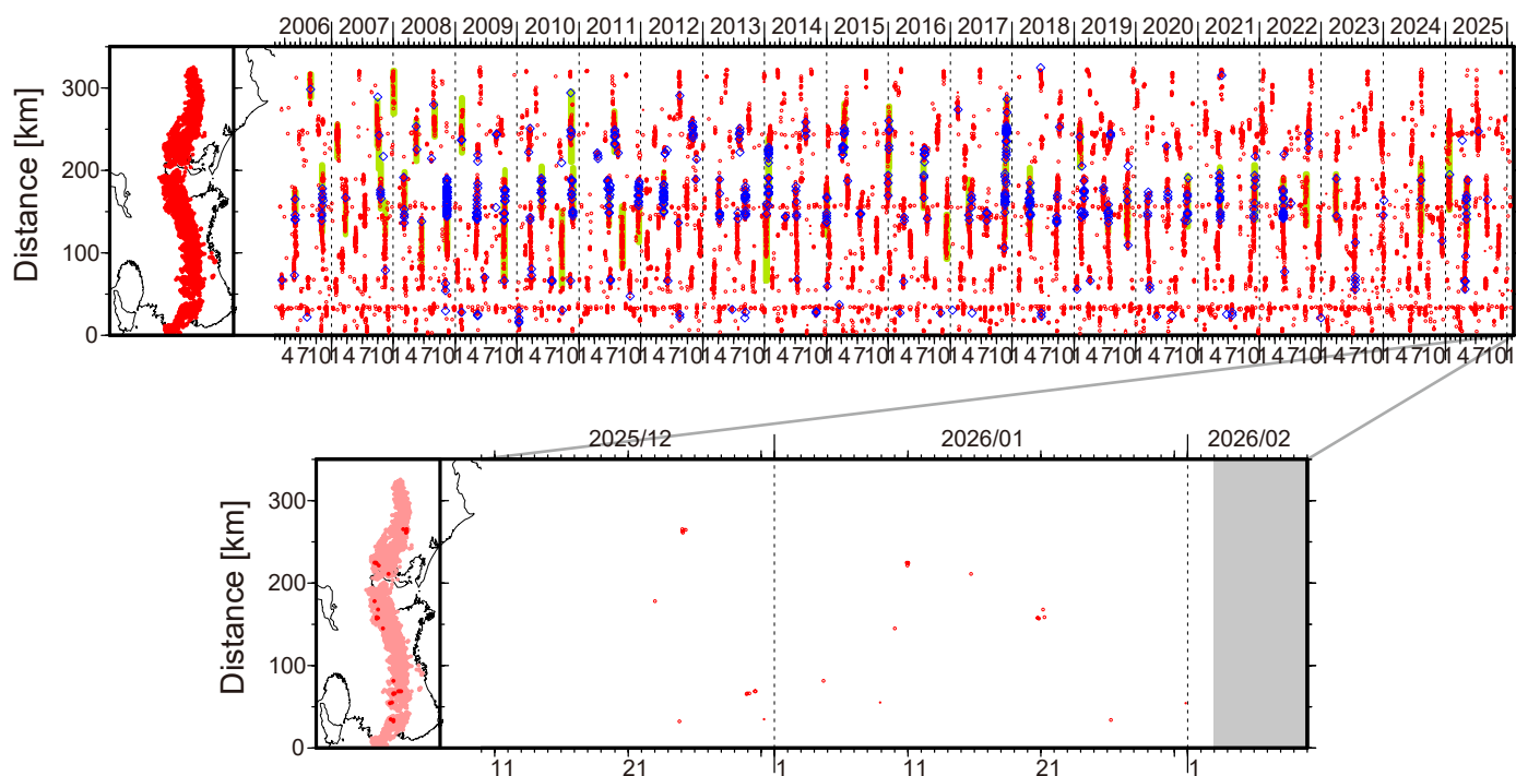
図 1. 紀伊半島・東海地域における 2006 年 2 月～2026 年 2 月 2 日までの深部低周波微動の時空間分布 (上図). 赤丸はエンベロープ相関・振幅ハイブリッド法 (Maeda and Obara, 2009) およびクラスタ処理 (Obara et al., 2010) によって 1 時間毎に自動処理された微動分布の重心である. 青菱形は周期 20 秒に卓越する超低周波地震 (Ito et al., 2007) である. 黄緑色の太線はこれまでに検出された短期的スロースリップイベント (SSE) を示す. 下図は 2026 年 1 月を中心とした期間の拡大図である. この期間において顕著な活動はとくにみられなかったものの, 1 月 10～11 日頃には愛知県西部において, 1 月 20～21 日頃には三重県北部において, それぞれごく小規模な活動がみられた.
