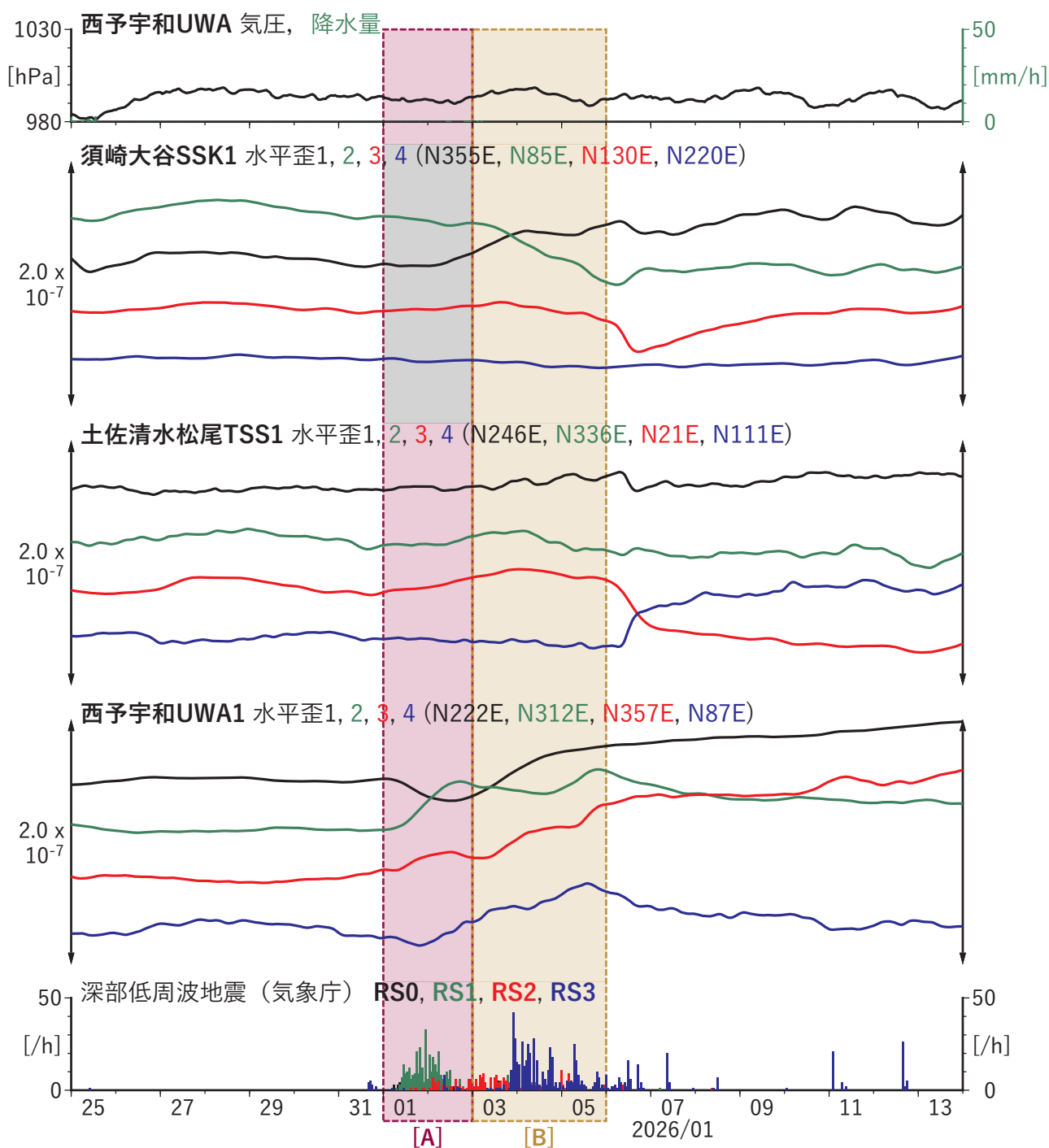
図5 歪・傾斜の時間変化(1) (2025/12/25 00:00–2026/01/14 00:00 (JST))
