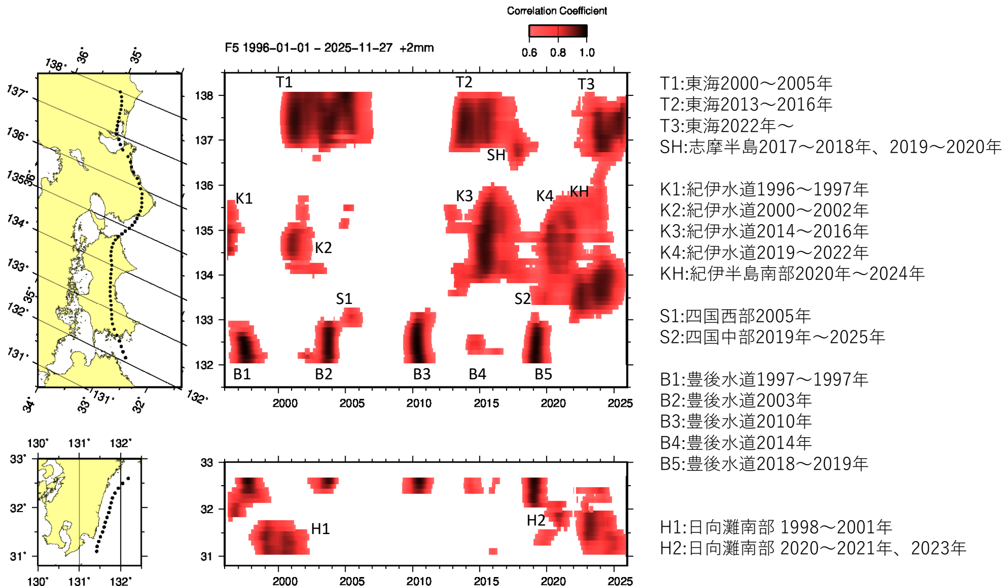
第1図 長期的スロースリップ客観検知図（1996年～2025年12月）
