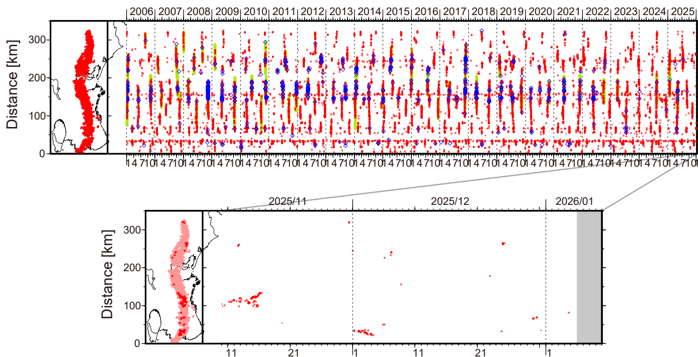
図 1. 紀伊半島・東海地域における 2006 年 1 月～2026 年 1 月 5 日までの深部低周波微動の時空間分布(上图). 赤丸はエンベロープ相関・振幅ハイブリッド法 (Maeda and Obara, 2009) およびクラスタ処理 (Obara et al., 2010) によって 1 時間毎に自動処理された微動分布の重心である. 青菱形は周期 20 秒に卓越する超低周波地震 (Ito et al., 2007) である. 黄緑色の太線はこれまでに検出された短期的スロースリップイベント (SSE) を示す. 下图は 2025 年 12 月を中心とした期間の拡大図である. 12 月 1 ～ 7 日頃には和歌山県中部において、やや活発な活動がみられた. やや西方向への活動域の移動がみられたのち、5 日頃から活動は低調となる一方、和歌山・奈良県境付近で若干の活動がみられた. 12 月 29 ～ 31 日頃には奈良県南部から和歌山県中部で小規模な活動がみられた. 12 月 7 日頃には愛知県西部において、12 月 25 日頃には愛知県東部において、それぞれごく小規模な活動がみられた.
