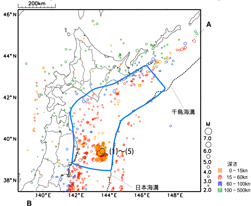
震央分布図（2025年11月1日～11月30日、M 2.0、深さ0～500km）
