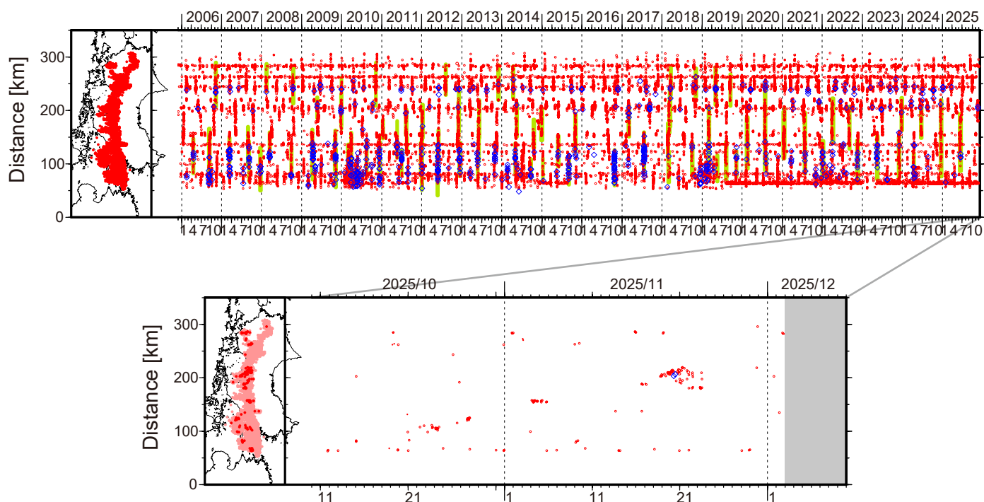
図 1. 四国における 2005 年 12 月～ 2025 年 12 月 2 日までの深部低周波微動の時空間分布（上図）．赤丸はエンベロープ相関・振幅ハイブリッド法 (Maeda and Obara, 2009) およびクラスタ処理 (Obara et al., 2010) によって 1 時間毎に自動処理された微動分布の重心である．青菱形は周期 20 秒に卓越する超低周波地震 (Ito et al., 2007) である．黄緑色太線は、これまでに検出された短期的スロースリップイベント (SSE) を示す．下図は 2025 年 11 月を中心とした期間の拡大図である．11 月 18 ～ 23 日頃には、愛媛県東部から中部においてやや活発な微動活動がみられた．この活動は愛媛県東部で開始した後、南東方向に活動域が拡大した後、20 日頃から東西両方向への活動域の拡大がみられた．11 月 4 ～ 5 日頃には愛媛県中部において、小規模な活動がみられた．11 月 1 日頃および 15 日頃には香川県付近において、11 月 16 ～ 17 日頃には愛媛県中部において、それぞれごく小規模な活動がみられた．
