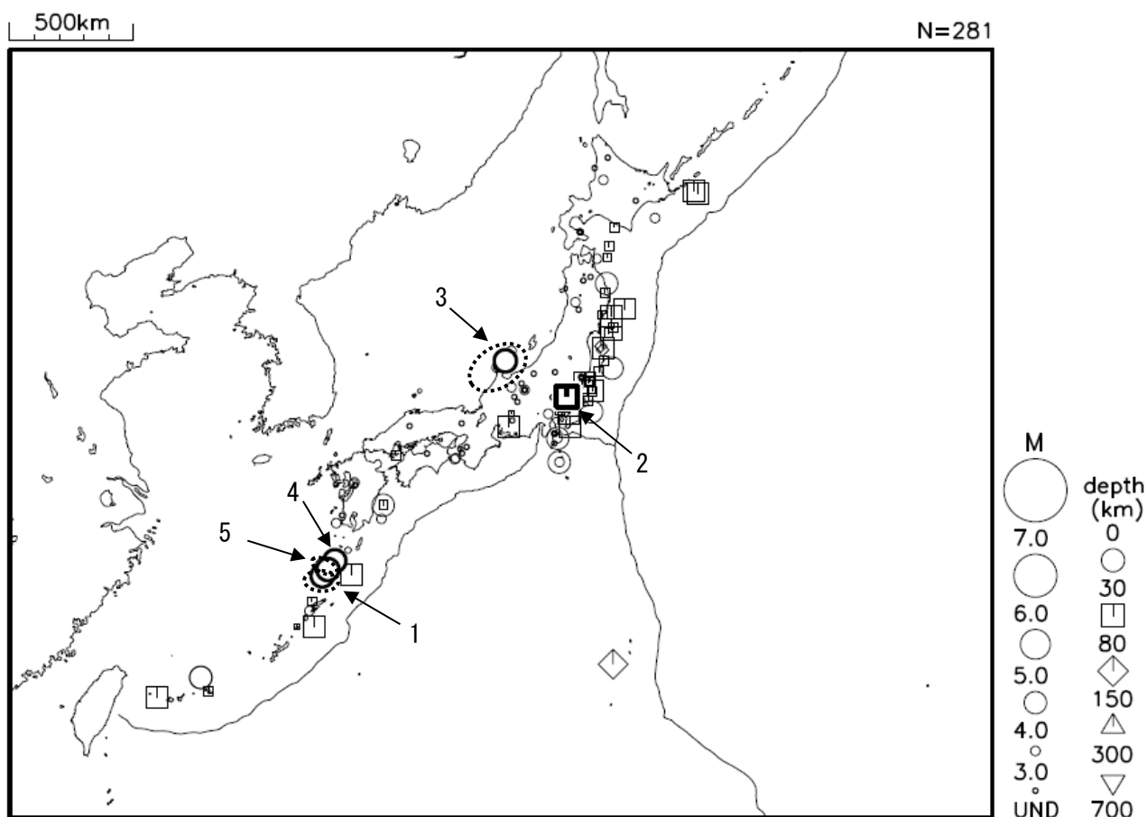
令和7年9月に震度1以上を観測した地震（図中の番号は、表の番号に対応）
