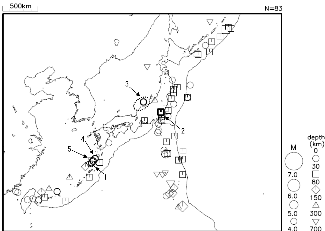
令和7年9月に発生した M4.0 以上の地震（図中の番号は、表の番号に対応）
