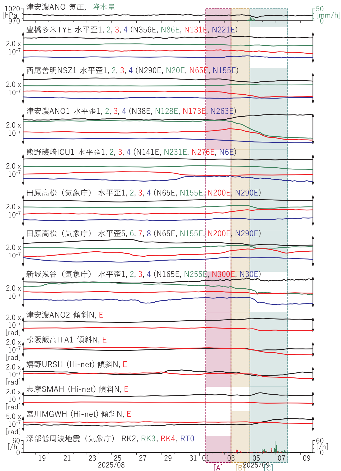
図2 東海・紀伊半島における歪・傾斜観測結果 (2025/08/18 00:00 - 2025/09/10 00:00 (JST))
