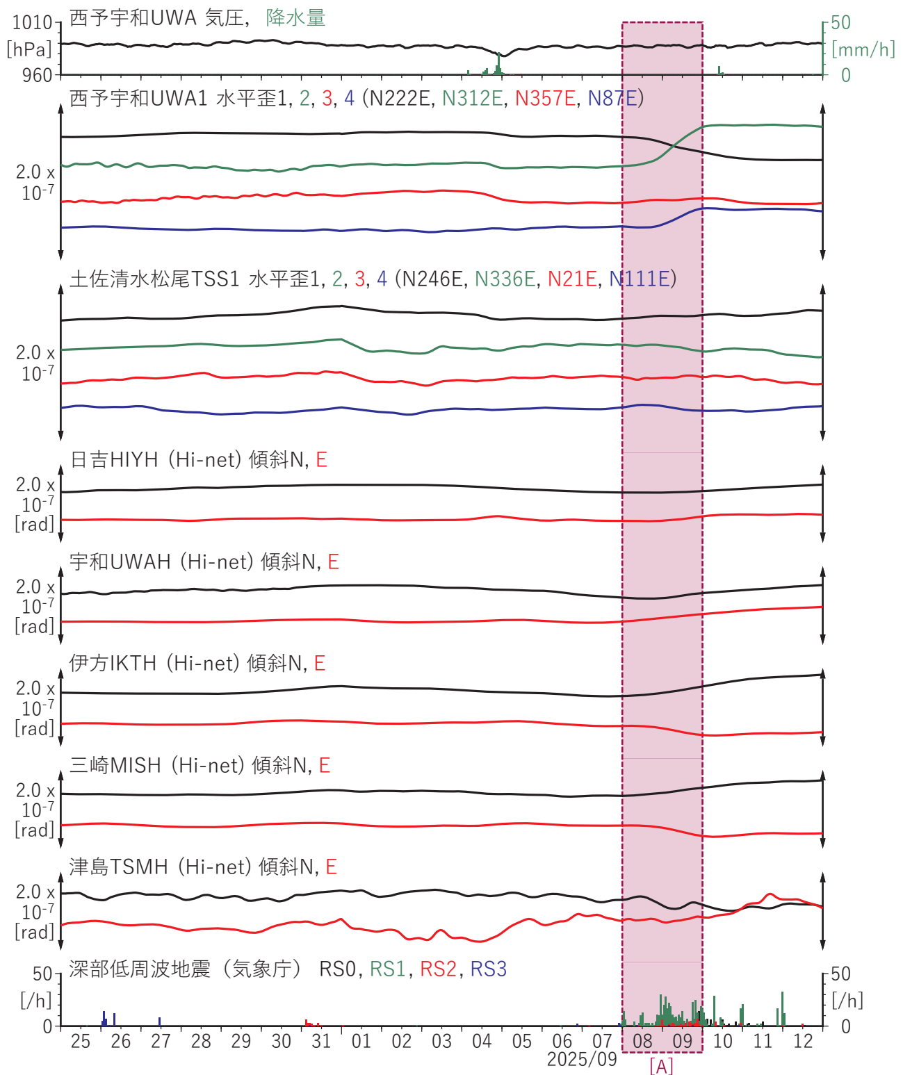
図7 四国地方における歪・傾斜観測結果 (2025/08/25 00:00 - 2025/09/13 00:00 (JST))
