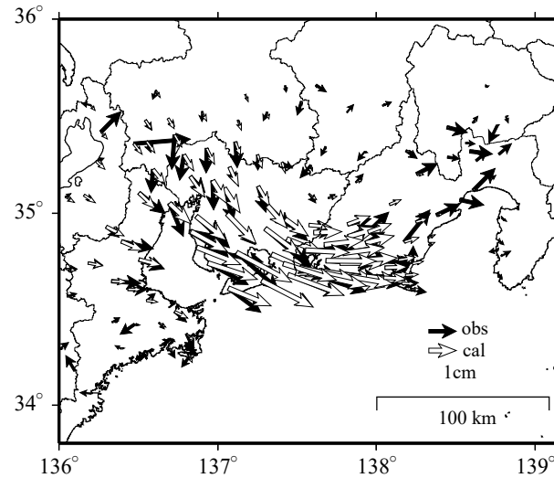
観測値(黒)と計算値(白)の比較 (2022-01-01/2025-09-09)
