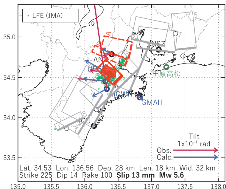
図5 2025/09/05-07の歪・傾斜変化（図2[C]）を説明する断層モデル。
