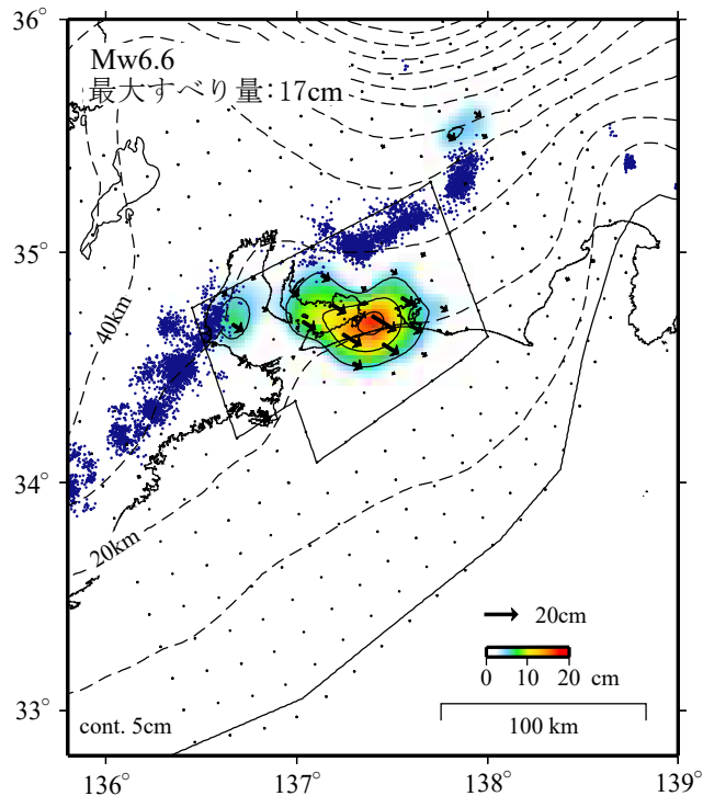
推定すべり分布 (2022-01-01/2025-09-09)
