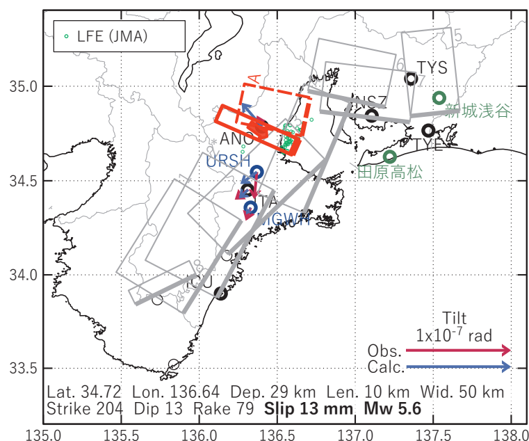
図4 2025/09/03PM-04の歪・傾斜変化（図2[B]）を説明する断層モデル。
