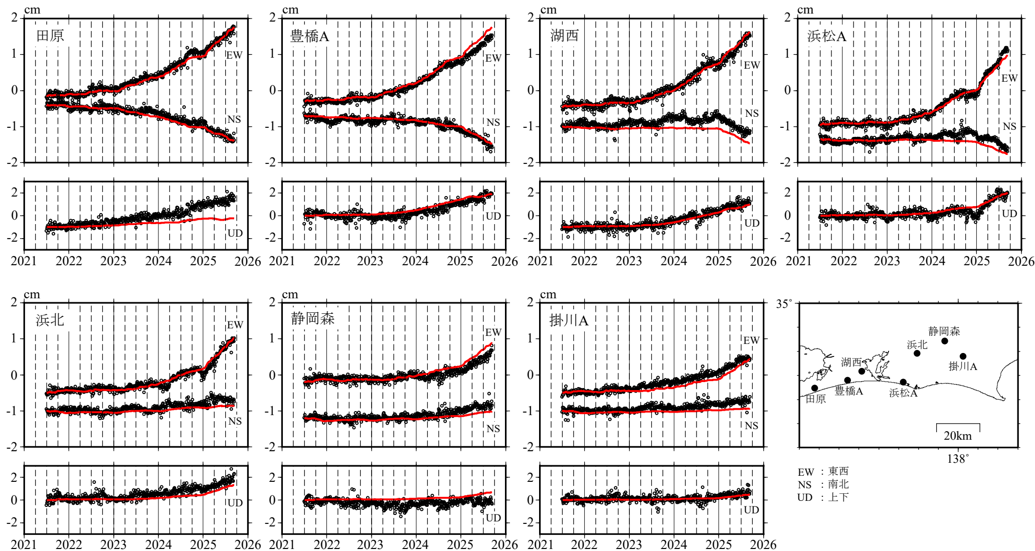
東海地域の観測点の座標時系列(黒丸)と計算値(赤線) 時間依存のインバージョン
