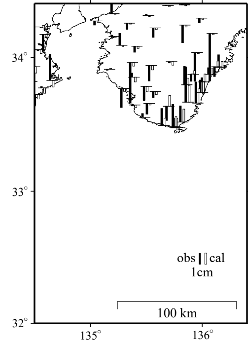
観測値(黒)と計算値(白)の比較 (2020-01-01/2025-09-17)
