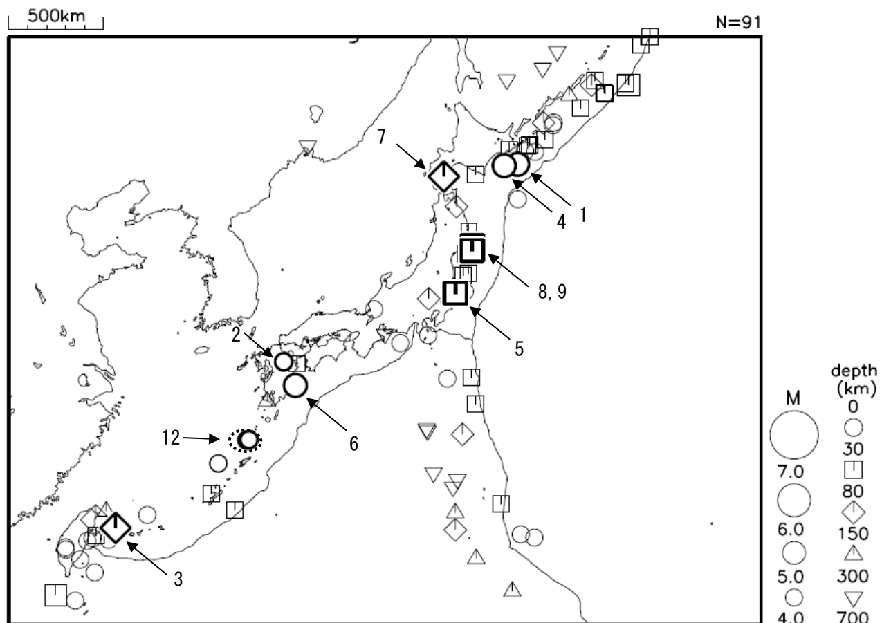
令和7年8月に発生した M4.0 以上の地震（図中の番号は、表の番号に対応）
