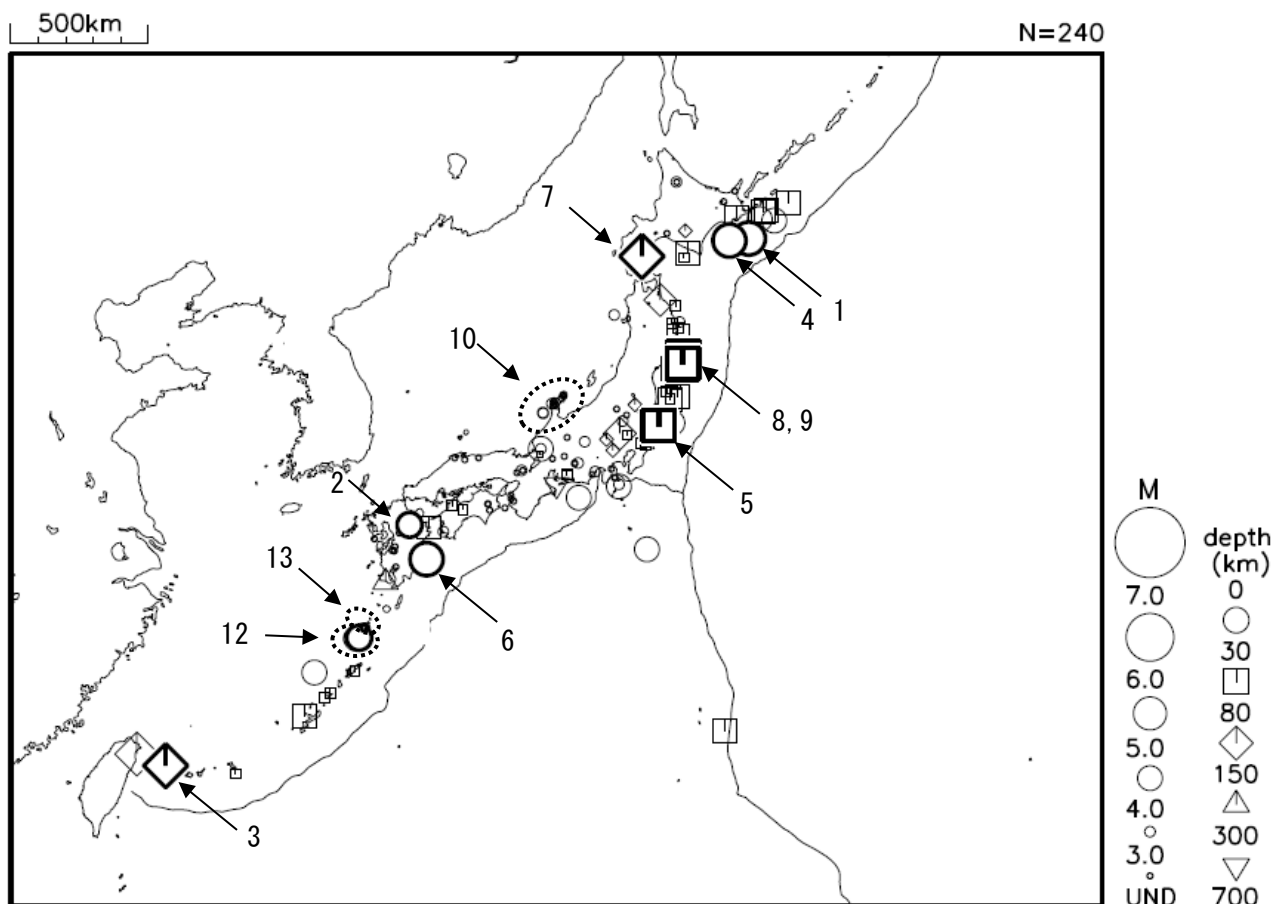
令和7年8月に震度1以上を観測した地震（図中の番号は、表の番号に対応）
