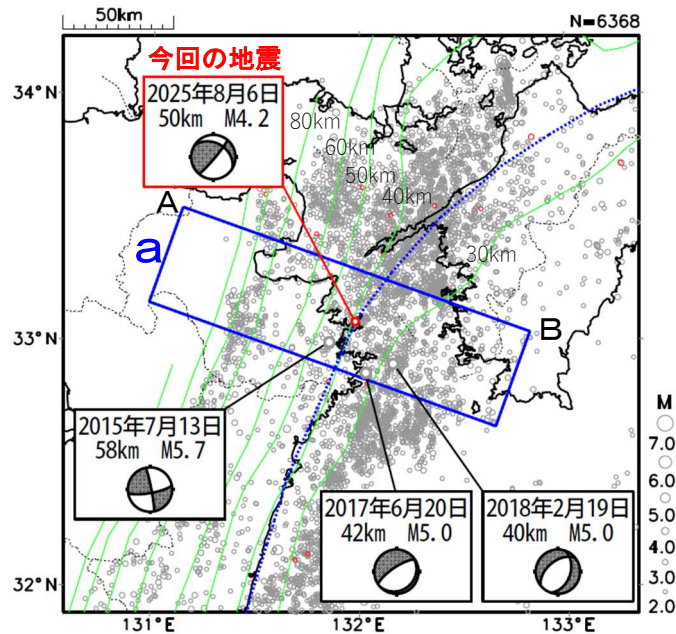
震央分布図 (1997年10月1日～2025年8月31日、深さ30～150km、 M \geq 2.0 ) 2025年8月の地震を赤色で表示
