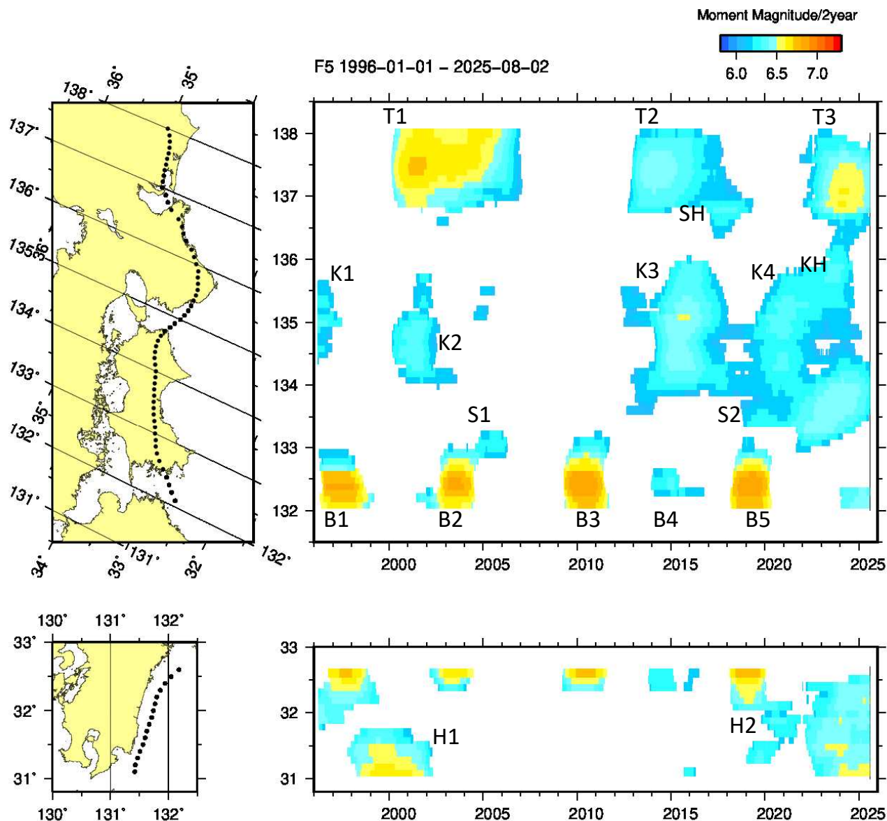
第2図 長期的スロースリップの規模分布（1996年～2025年8月） 2年間あたりの変化量から推定したモーメントマグニチュード。
