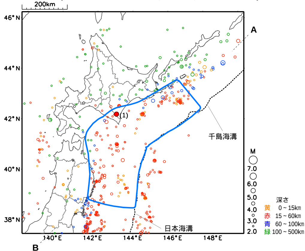
震央分布図（2025年7月1日～7月31日、M 2.0、深さ0～500km）
