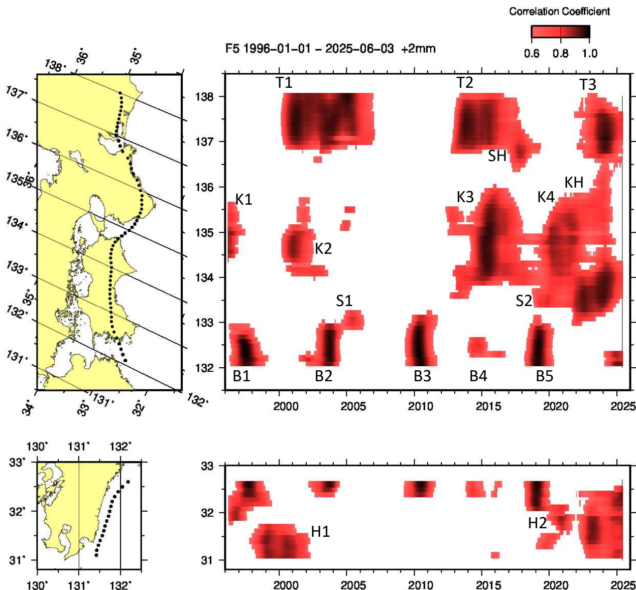
第1図 長期的スロースリップ客観検知図（1996年～2025年6月）
