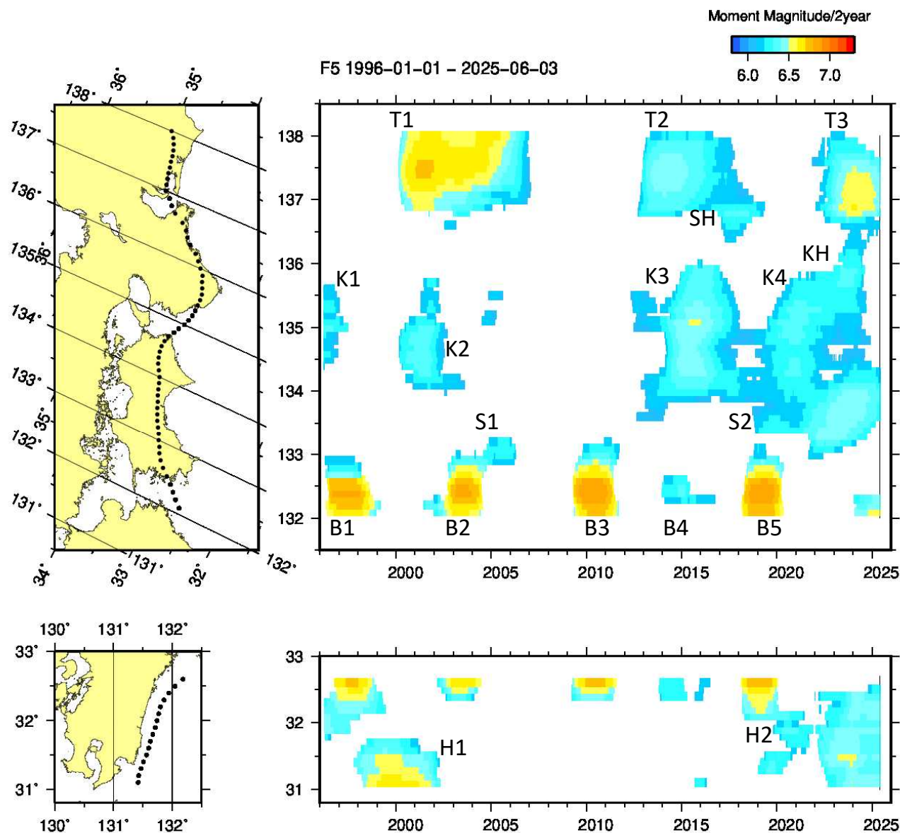
第2図 長期的スロースリップの規模分布（1996年～2025年6月） 2年間あたりの変化量から推定したモーメントマグニチュード。
