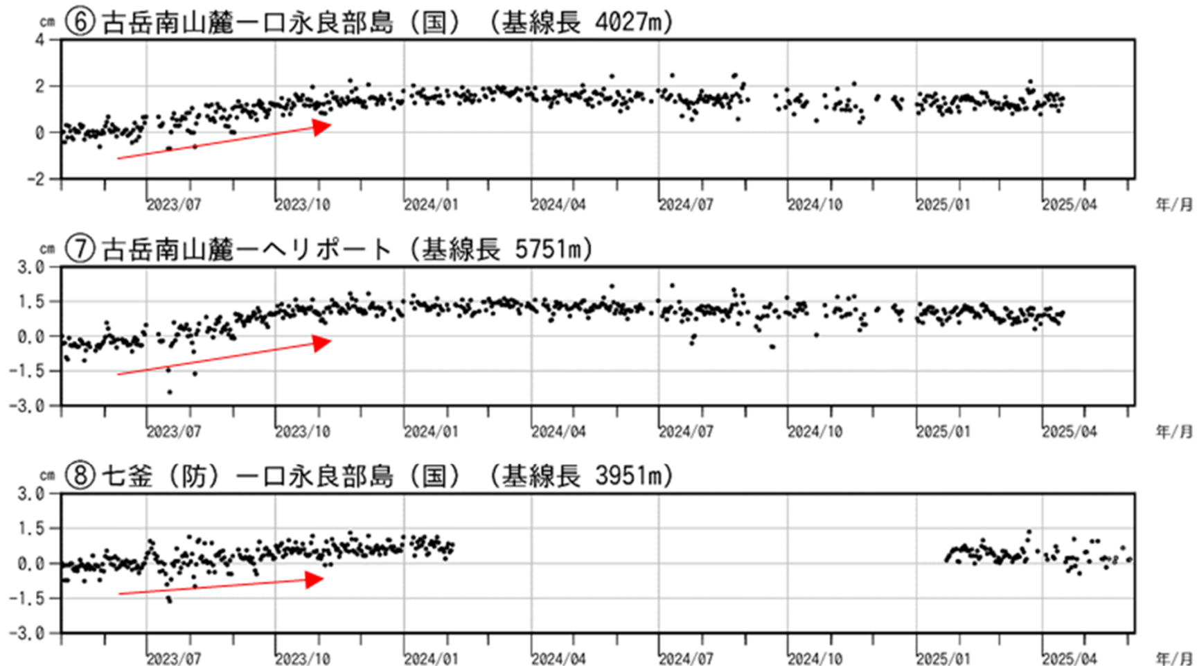
図2 口永良部島 GNSS連続観測による基線長変化 (2023年5月1日～2025年6月10日)
