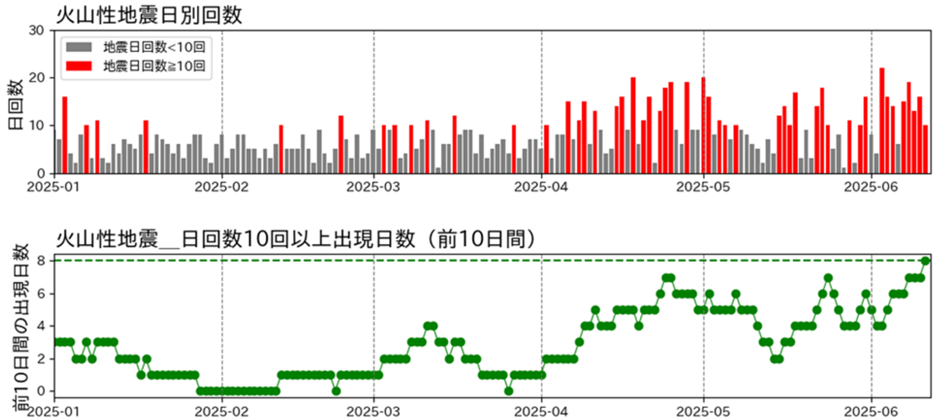
図1 口永良部島 火山性地震の日別回数と日回数10回以上出現日数 (2025年1月1日～6月11日21時)
