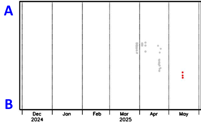
領域a内の時空間分布図(A-B投影) (2024年11月～2025年5月)
