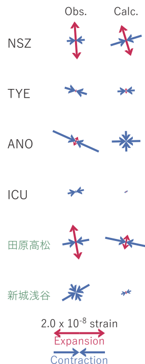
図8 2025/05/09PM-14の歪・傾斜変化（図3[E]）を説明する断層モデル。
