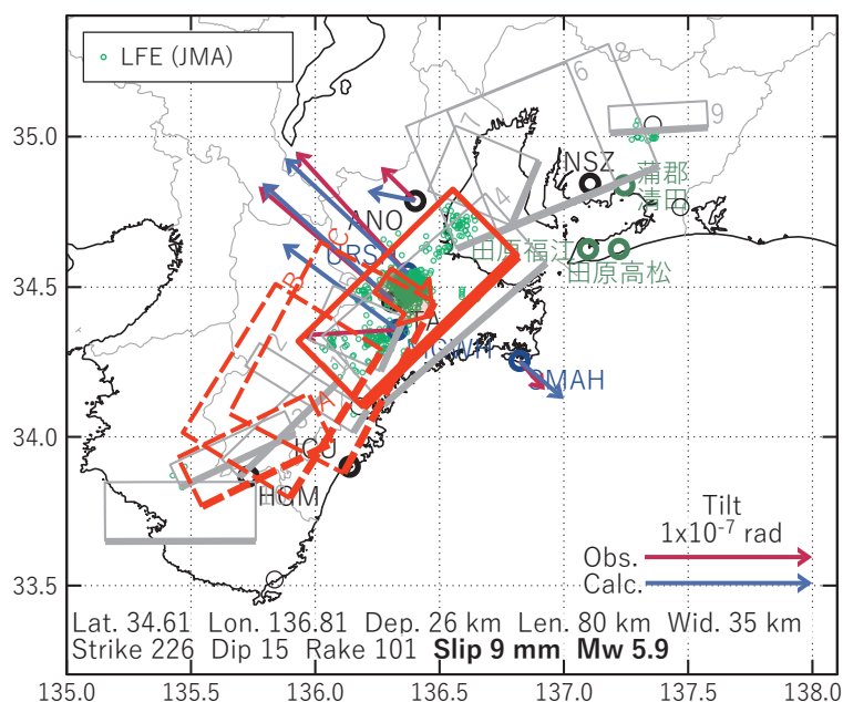
図7 2025/05/05PM-09AMの歪・傾斜変化(図3[D])を説明する断層モデル。
