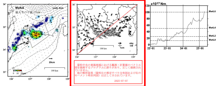
GNSSデータから推定された東海地域の長期的ゆっくりすべり（暫定） 推定すべり分布 (2022-01-01/2025-04-21) 観測値（黒）と計算値（白）の比較 (2022-01-01/2025-04-21) モーメント* 時系列（試算）
