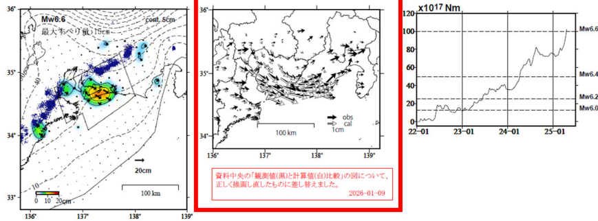
GNSSデータから推定された東海地域の長期的ゆっくりすべり（暫定） 推定すべり分布 (2022-01-01/2025-04-21) 観測値（黒）と計算値（白）の比較 (2022-01-01/2025-04-21) モーメント* 時系列（試算）
