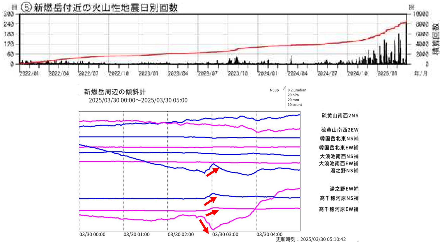
図1 霧島山（新燃岳）日別地震回数及び傾斜計による地殻変動の状況
