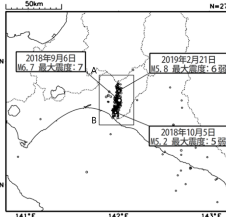
2018. 9. 6-2021. 9. 6 M ≥ 3. 0
