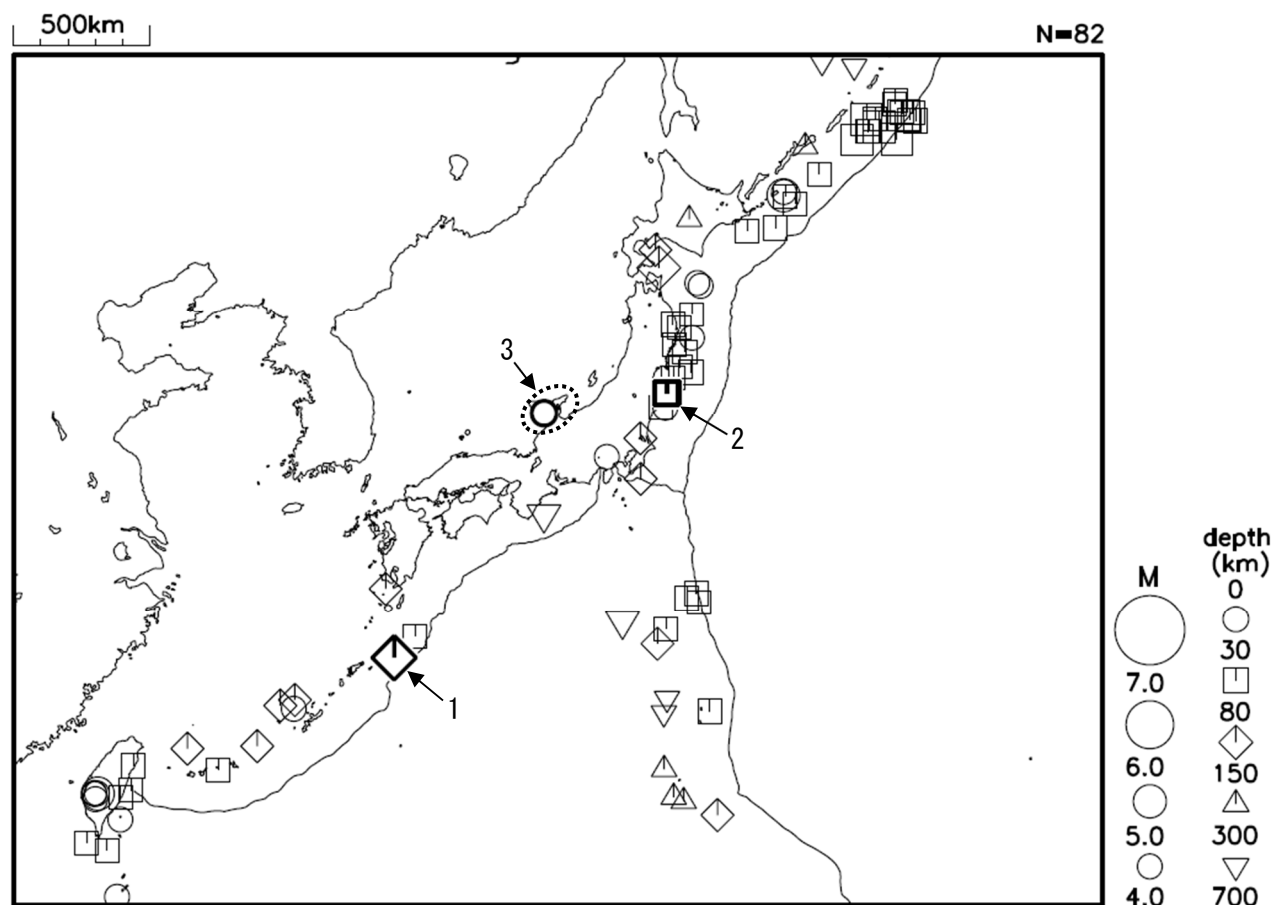
令和7年2月に発生した M4.0 以上の地震（図中の番号は、表の番号に対応）
