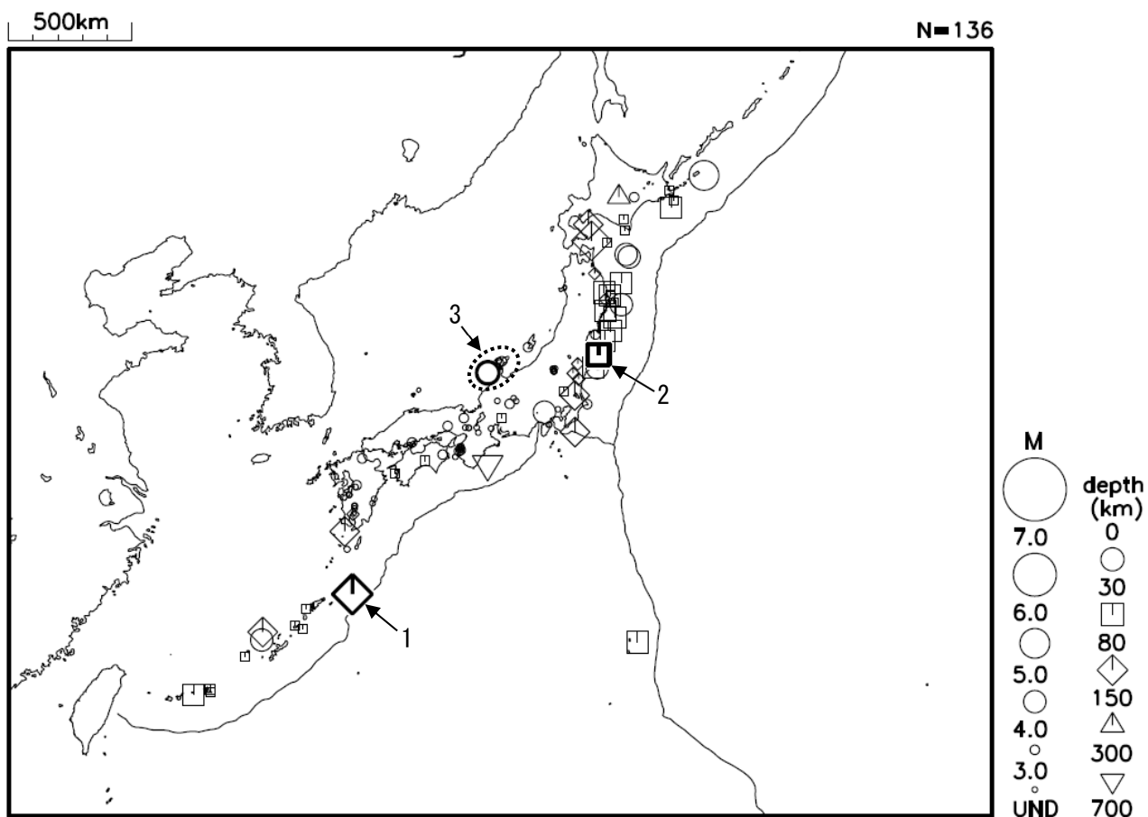
令和7年2月に震度1以上を観測した地震（図中の番号は、表の番号に対応）
