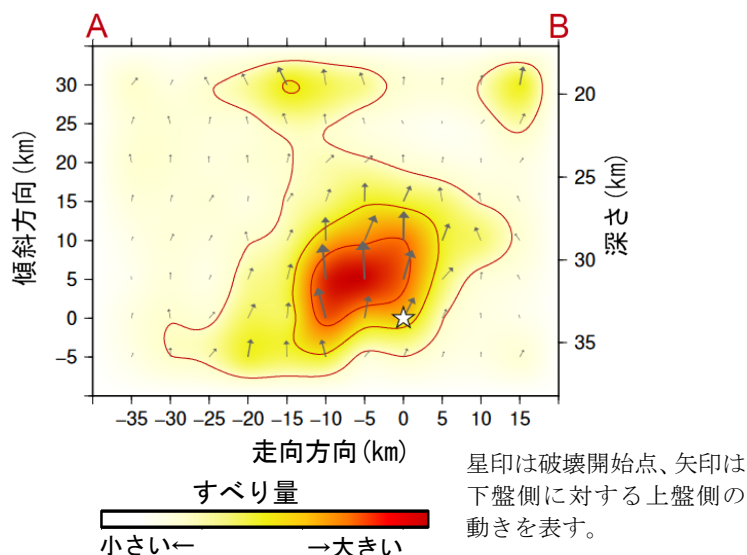
図 2-7 断層面上でのすべり量分布
