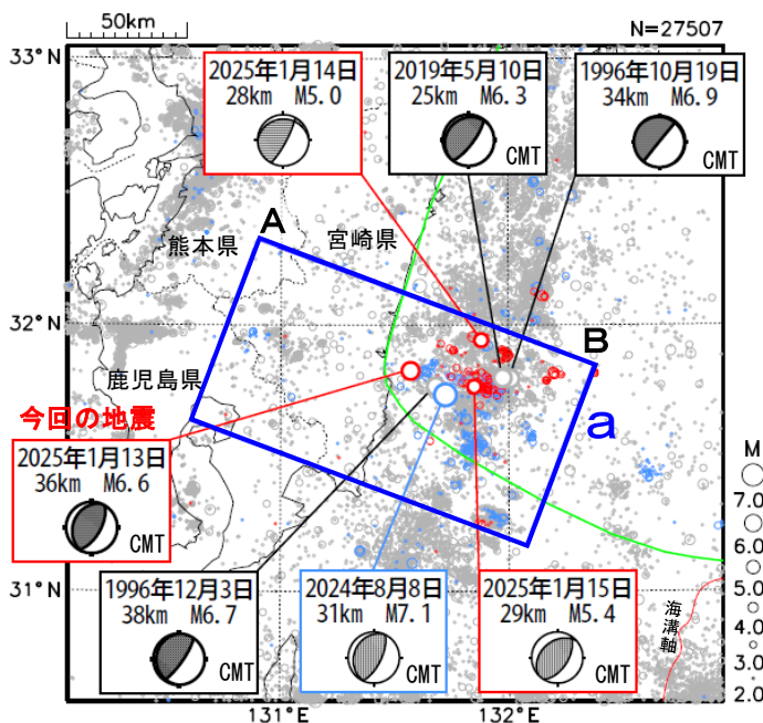
図 2-1 震央分布図 (1994 年 10 月 1 日～2025 年 1 月 31 日 深さ 0～100km、M≥2.0)
