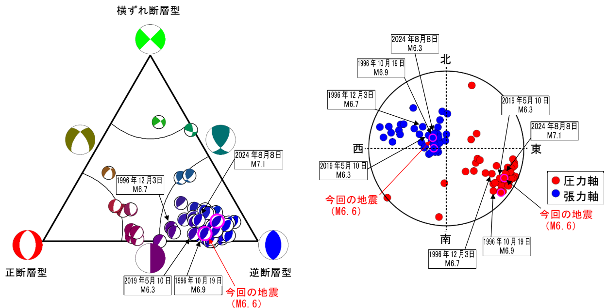
図2-5 図2-4の領域c内の地震の発震機構の型の分布（左）及び発震機構の圧力軸及び張力軸の方位分布（右）
