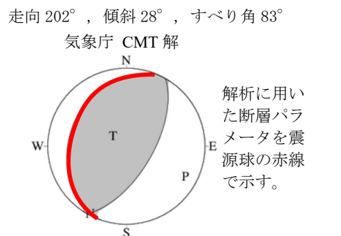
図 2-9 解析に用いた断層パラメータ
