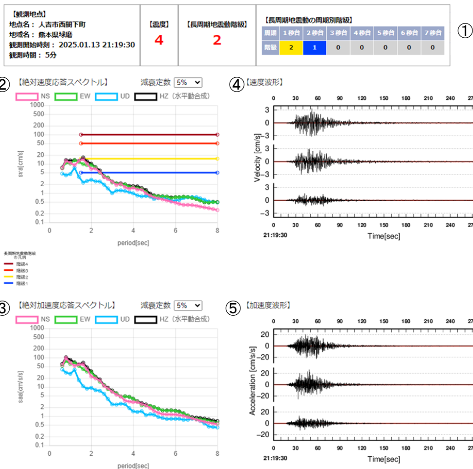
図４－２ 人吉市西間下町で観測した波形、絶対速度応答スペクトル及び絶対加速度応答スペクトル (ただし、速度波形、加速度波形は21時19分30秒からの5分間を表示)
