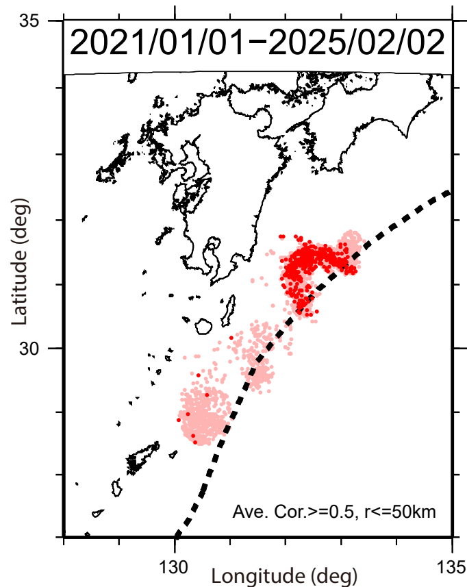
第1図. 2021年1月1日から2025年2月2日までの期間内に波形相関解析 [Asano et al. (2015)] によって検出された超低周波イベントの震央分布. 検出イベントを防災科研の手動または自動検測震源と照合して通常の地震を除去した後に、それ以外を超低周波イベントとして桃色（2024年12月31日以前）、および赤色（2025年1月1日以降）の点でそれぞれ示す。
