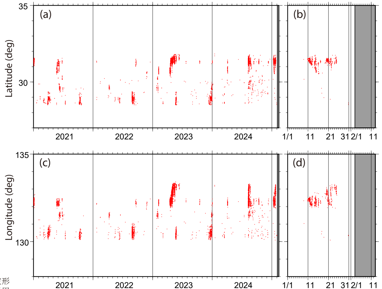
第2図. 第1図と同じ期間内に検出された超低周波イベントの時空間分布. 超低周波イベントを赤色の点で示す. (a)および(b)に緯度分布の、(c)および(d)に経度分布の時間変化をそれぞれ示す. また、(a)および(c)に2021年1月1日以降、(b)および(d)には2025年1月1日以降の分布をそれぞれ示す。
