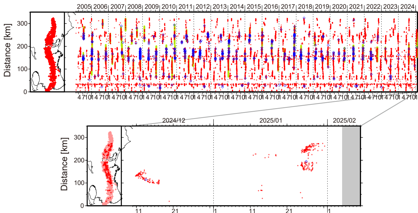
図 1. 紀伊半島・東海地域における 2005 年 2 月～2025 年 2 月 4 日までの深部低周波微動の時空間分布（上図）．赤丸はエンベロープ相関・振幅ハイブリッド法 (Maeda and Obara, 2009) およびクラスタ処理 (Obara et al., 2010) によって 1 時間毎に自動処理された微動分布の重心である．青菱形は周期 20 秒に卓越する超低周波地震 (Ito et al., 2007) である．黄緑色の太線はこれまでに検出された短期的スロースリップイベント (SSE) を示す．下図は 2025 年 1 月を中心とした期間の拡大図である．1 月 24 ～ 31 日頃には三重県北部から愛知県東部において、活発な微動活動がみられた．この活動は愛知県西部および三重県北部で開始したのち、それぞれ東方向および西方向への拡大がややみられた．愛知県側および三重県側では、それぞれ 30 日頃および 28 日頃から活動が低調となった．この活動に際し、傾斜変動から短期的 SSE の断層モデルも推定されている．1 月 13 ～ 14 日頃には奈良県南部から和歌山県中部において、1 月 17 ～ 18 日頃には愛知県西部において、それぞれごく小規模な活動がみられた．
