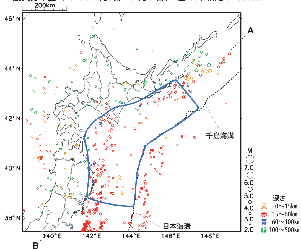
震央分布図（2024年12月1日～12月31日、 M \geq 2.0 、深さ0～500km）
