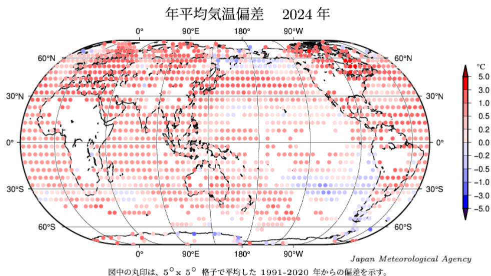
図2 2024年の年平均気温偏差の分布図（速報）
