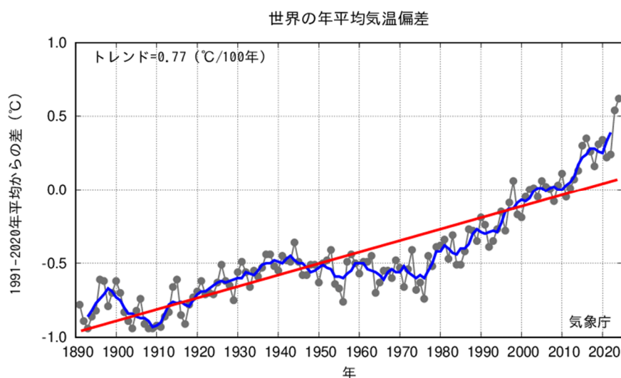
図 1 世界の年平均気温偏差の経年変化（1891～2024 年、速報）
