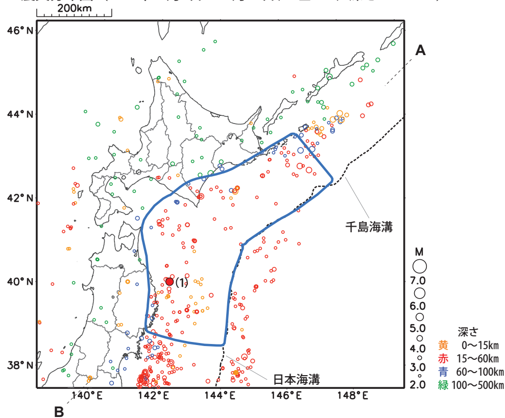
震央分布図（2024年10月1日～10月31日、 M \geq 2.0 、深さ0～500km）
