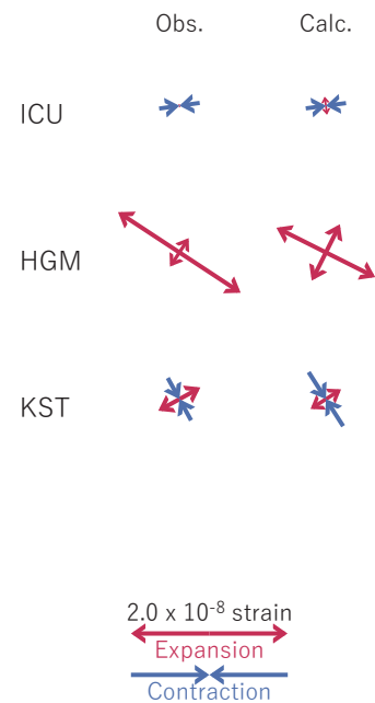
図6 2024/06/15-17の歪・傾斜変化(図5[A])を説明する断層モデル。
