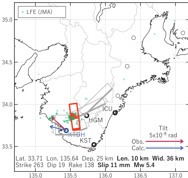
図6 2024/06/15-17の歪・傾斜変化(図5[A])を説明する断層モデル。
