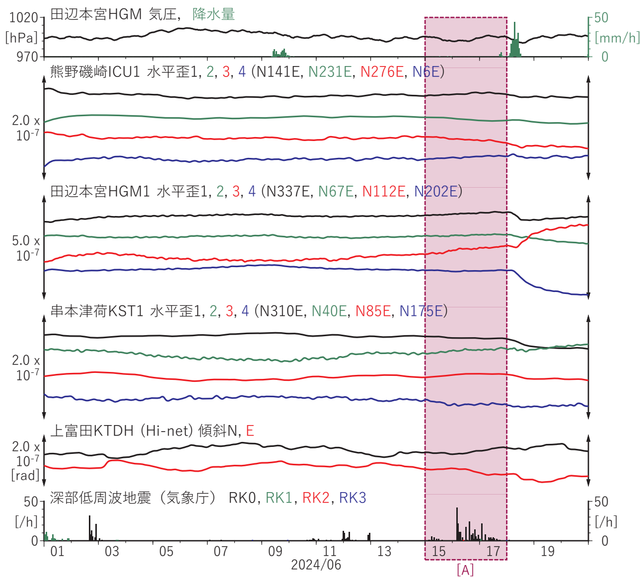
図5 紀伊半島における歪・傾斜観測結果 (2024/06/01 00:00 - 2024/06/21 00:00 (JST))
