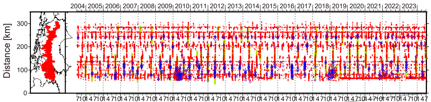
図 1. 四国における 2004 年 7 月～2024 年 7 月 2 日までの深部低周波微動の時空間分布 (上図). 赤丸はエンベロープ相関・振幅ハイブリッド法 (Maeda and Obara, 2009) およびクラスタ処理 (Obara et al., 2010) によって 1 時間毎に自動処理された微動分布の重心である. 青菱形は
