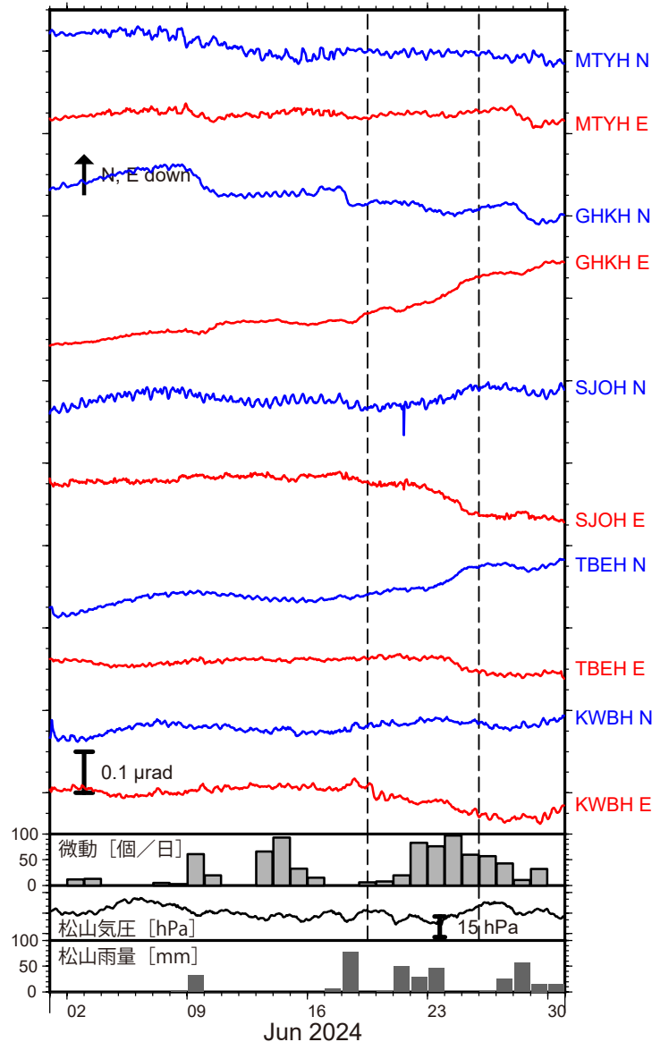
図 1: 2024 年 6 月 1 日～6 月 30 日の傾斜時系列。上方向への変化が北・東下がりの傾斜変動を表し、BAYTAP-G により潮汐・気圧応答成分を除去した。6 月 19 日 12 時～6 月 25 日の傾斜変化ベクトルを図 2 に示す。四国中部での微動活動度・気象庁松山観測点の気圧・雨量をあわせて示す。
