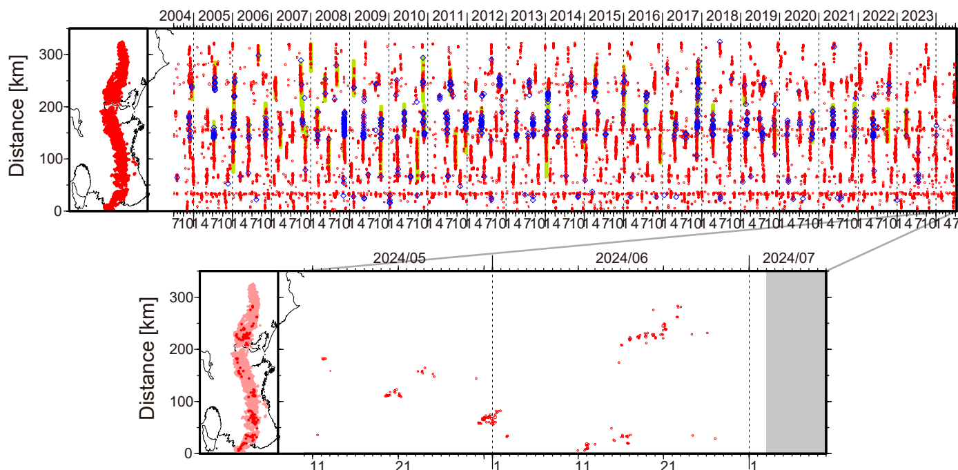
図 1. 紀伊半島・東海地域における 2004 年 7 月～2024 年 7 月 2 日までの深部低周波微動の時空間分布（上図）。赤丸はエンベロップ相関・振幅ハイブリッド法 (Maeda and Obara, 2009) およびクラスタ処理 (Obara et al., 2010) によって 1 時間毎に自動処理された微動分布の重心である。青菱形は周期 20 秒に卓越する超低周波地震 (Ito et al., 2007) である。黄緑色の太線はこれまでに検出された短期的スロースリップイベント (SSE) を示す。下図は 2024 年 6 月を中心とした期間の拡大図である。5 月 30 日～6 月 2 日頃に奈良・和歌山県境付近から和歌山県中部においてやや活発な微動活動がみられた。この活動は奈良・和歌山県境付近で開始し、やや北方向への活動域の拡大がみられたのち、6 月 2 日頃には和歌山県中部で活動がみられた。6 月 10～12 日頃および 6 月 14～17 日頃にはそれぞれ和歌山県中部において、小規模な活動がみられた。6 月 15～23 日頃には三重県北部から愛知・長野県境付近で小規模な活動がみられた。この活動では 15 日頃に三重県北部で微動活動がみられたのち、16 日頃から愛知県側で活動が開始した。20 日頃からは東方向に活動域の移動がみられ、22～23 日頃には愛知・長野付近で活動がみられた。
