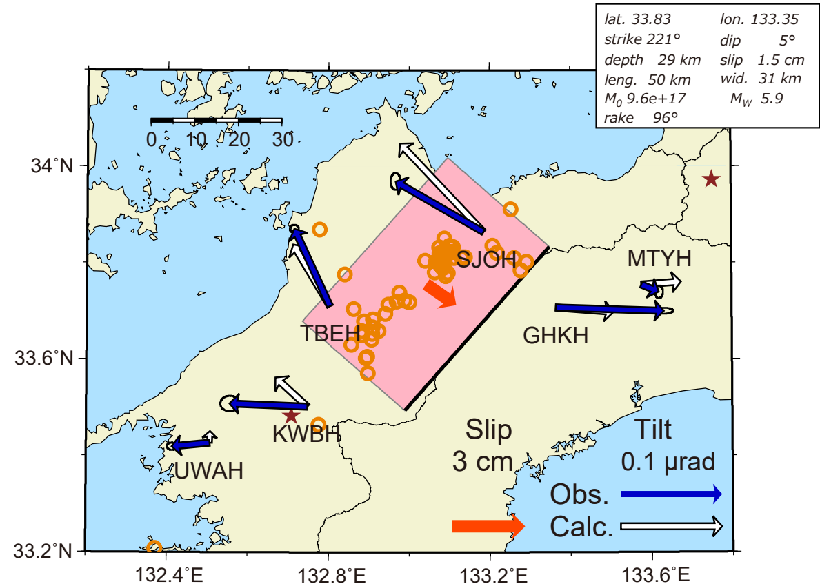
図 2: 6 月 19 日 12 時～6 月 25 日に観測された傾斜変化ベクトル (青矢印)、推定されたスロースリップイベントの断層モデル (赤矩形・矢印)、モデルから計算される傾斜変化ベクトル (白抜き矢印) を示す。1 時間ごとの微動エネルギーの重心位置 (橙丸)、深部超低周波地震 (茶星印) もあわせて示す。すべり角はプレート相対運動方向に固定している。
