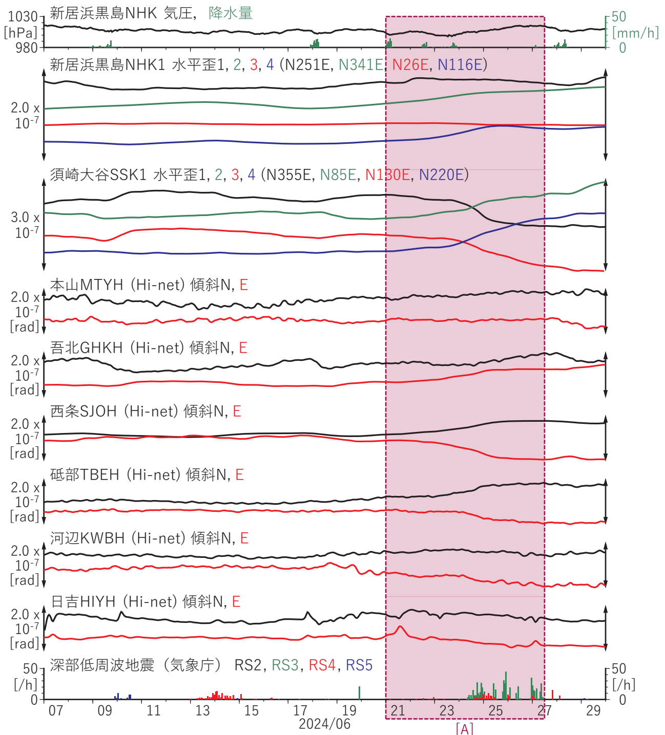
図12 四国における歪・傾斜観測結果 (2024/06/02 00:00 - 2024/06/31 00:00 (JST))
