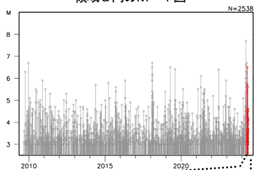
領域a内の回数積算及びM-T図 (4月1日～5月31日)
