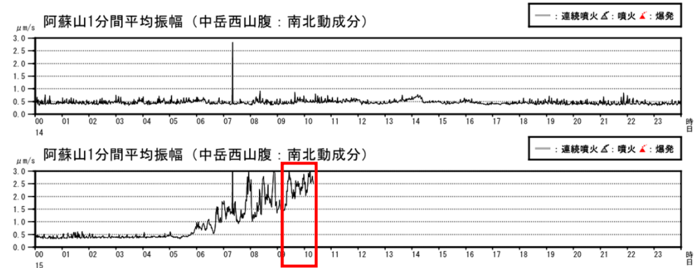
図 阿蘇山の火山性微動の1分間平均振幅の推移 （上段：2024年5月14日、下段：2024年5月15日 10時過ぎまで） 2024年5月15日09時過ぎから火山性微動の振幅が 1.5マイクロメートル毎秒を超えてやや大きい状態で継続しています。
