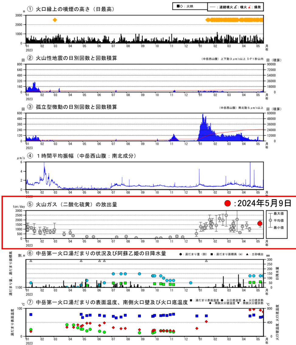
図 阿蘇山の火山活動経過図（2023年1月1日～2024年5月15日） 2024年5月9日に実施した現地調査では、火山ガス（二酸化硫黄）の放出量が 1日あたり1600トンと、やや多い状態でした。
