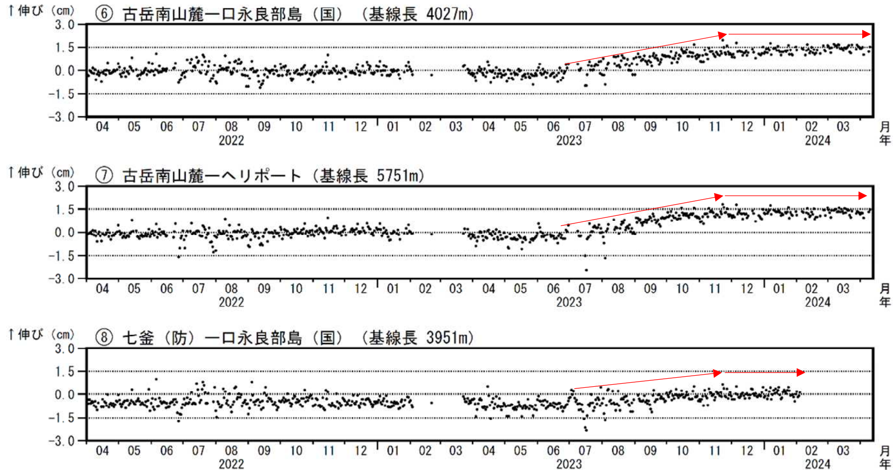
図2 口永良部島 GNSS連続観測による基線長変化 (2022年4月～2024年4月12日)
