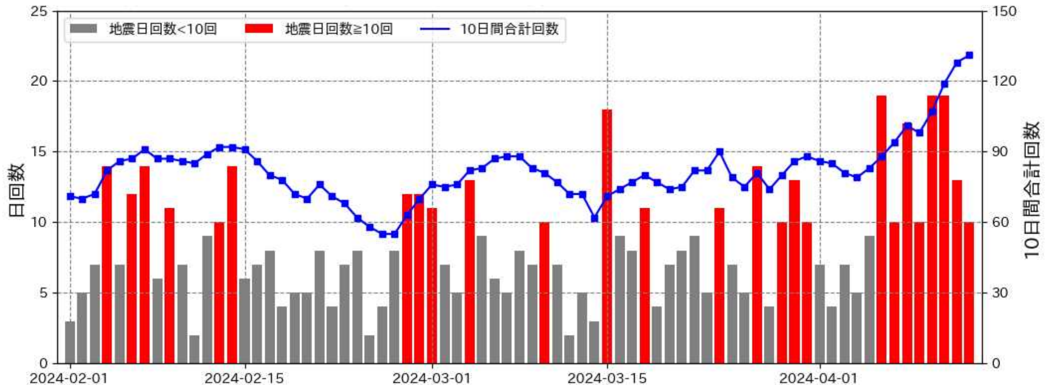
図1 口永良部島 火山性地震の日別回数と10日間合計回数 (2024年2月1日～4月13日12時30分まで)
