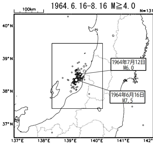
1964年新潟地震 (M7.5, 最大震度5)
