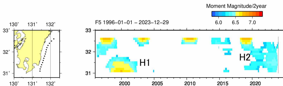
第2図 長期的スロースリップの規模分布（1996年から2023年12月） 2年間あたりの変化量から推定したモーメントマグニチュード。地域略号は第1図と同じ。
