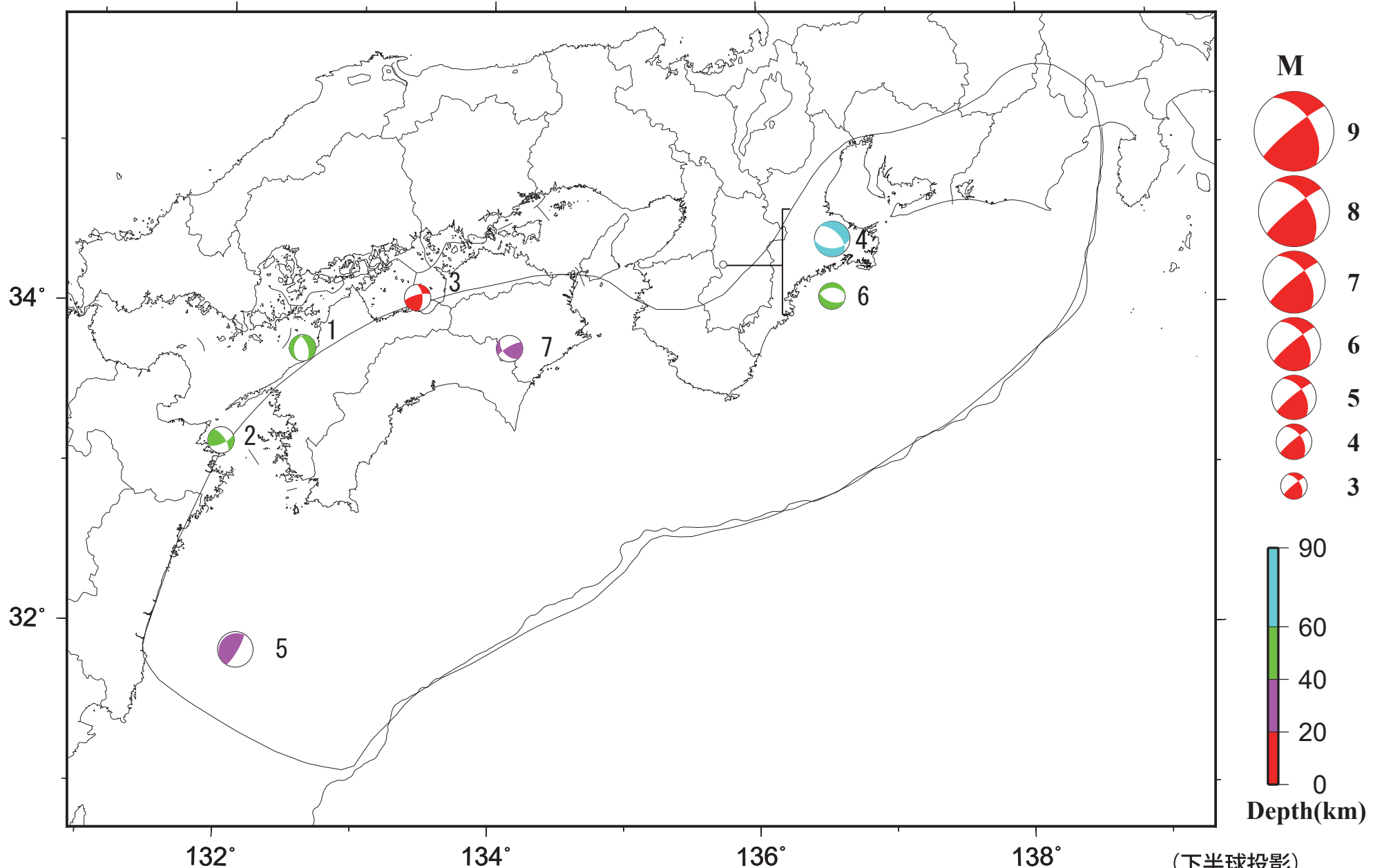
図中には M \geq 3.2 、 0 \text{ km} \leq \text{深さ} \leq 90 \text{ km} の地震についての初動発震機構解を示す。数字は次頁の発震機構解を示す。
