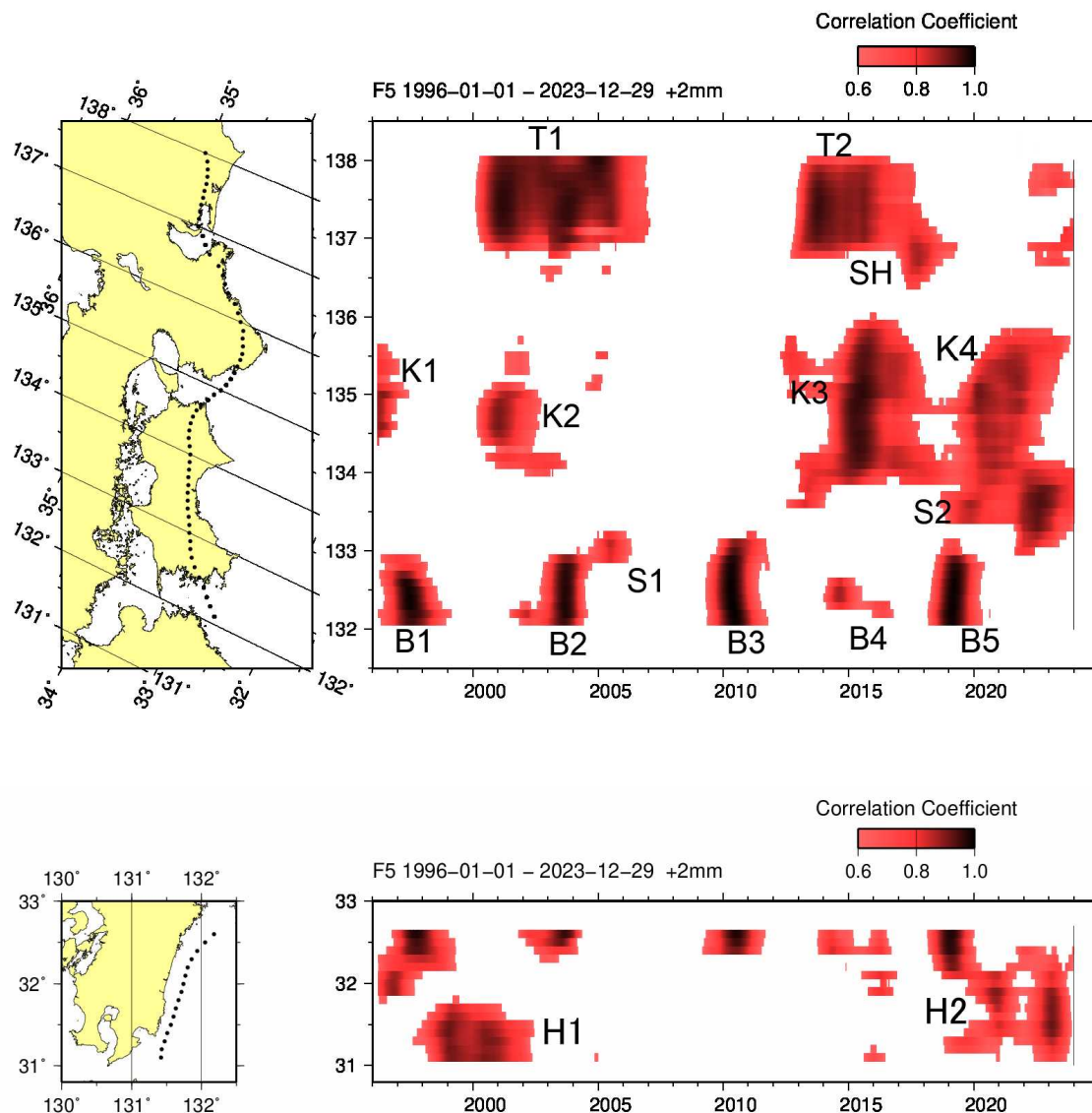
第1図 長期的スロースリップ客観検知図（1996年から2023年12月）
