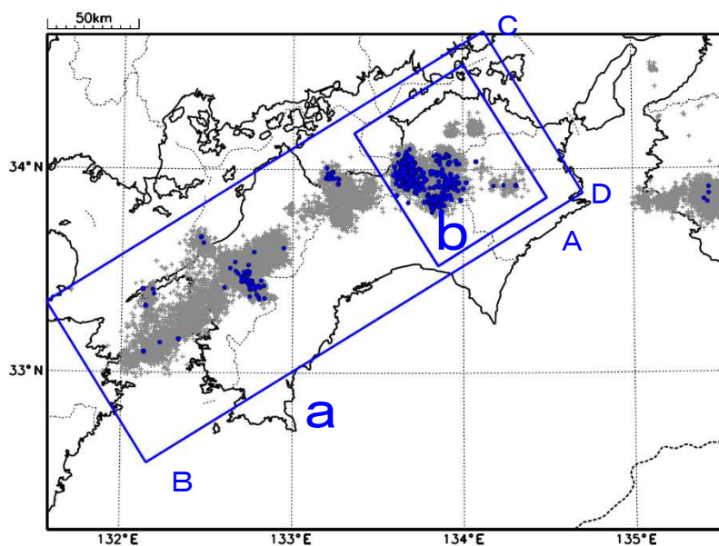
震央分布図(2018年4月1日~2024年2月5日、 深さ0~60km、Mすべて) 灰:2018年4月1日~2024年1月24日、 青:2024年1月25日以降
