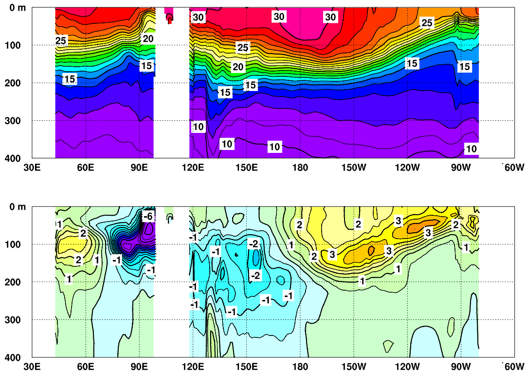
図5 2023年11月のインド洋から太平洋の赤道に沿った水温（上）及び平年偏差（下）の断面図
