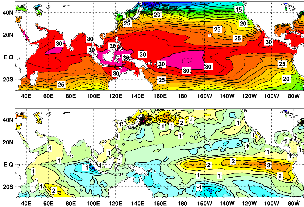
図4 2023年11月の海面水温図（上）及び平年偏差図（下）
