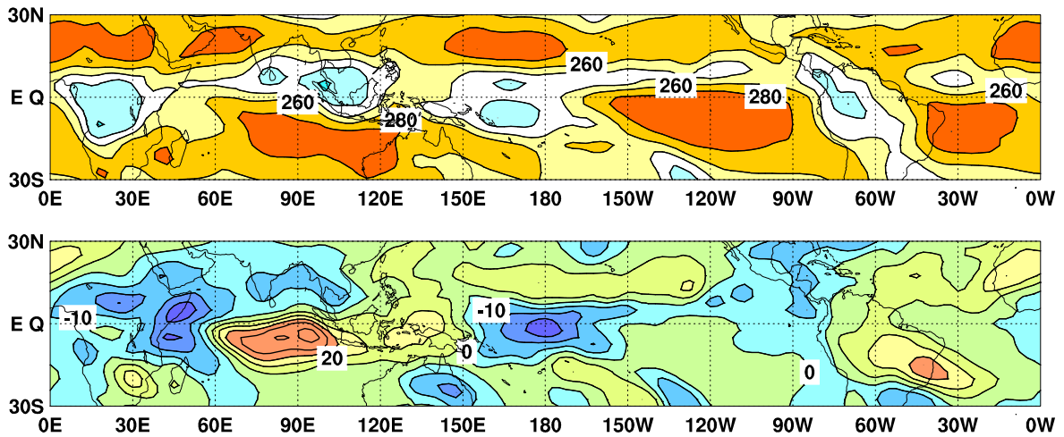
図9 外向き長波放射量 (OLR) (上) 及び年偏差 (下) の分布図 (2023年11月)
