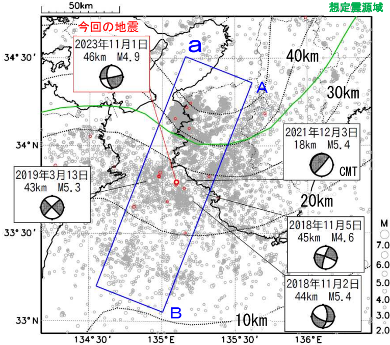
震央分布図 (1997年10月1日～2023年11月30日、 深さ0～80km、 M \geq 2.0 ) 2023年11月1日以降の地震を赤く表示
