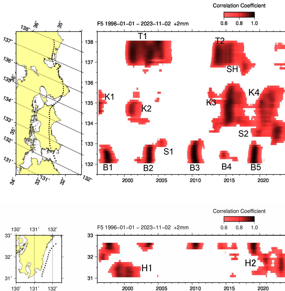
第1図 長期的スロースリップ客観検知図（1996年から2023年11月）
