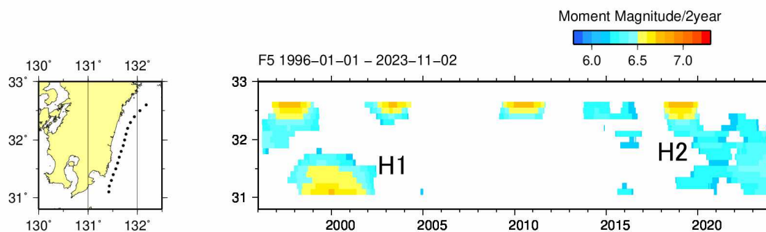
第2図 長期的スロースリップの規模分布（1996年から2023年11月） 2年間あたりの変化量から推定したモーメントマグニチュード。地域略号は第1図と同じ。
