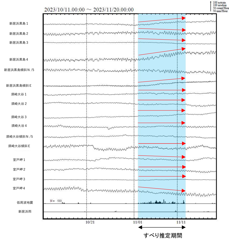
新居浜黒島、須崎大谷及び室戸岬は産業技術総合研究所のひずみ・傾斜計である。
