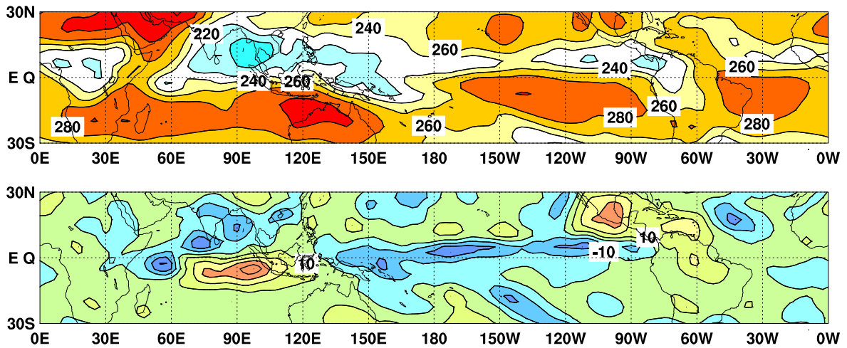
図9 外向き長波放射量 (OLR) (上) 及び年偏差 (下) の分布図 (2023年9月)
