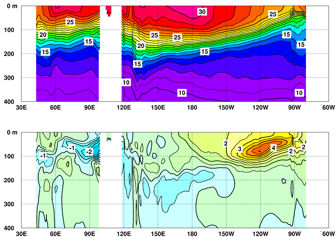
図5 2023年9月のインド洋から太平洋の赤道に沿った水温（上）及び平年偏差（下）の断面図
