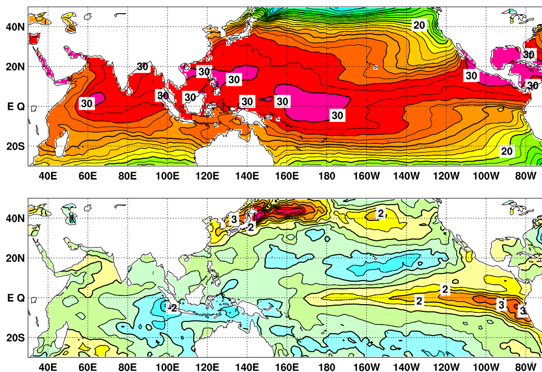
図4 2023年9月の海面水温図（上）及び平年偏差図（下）
