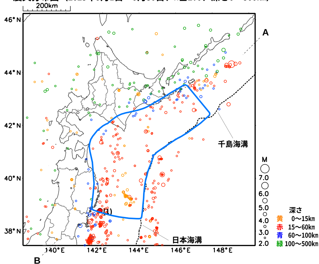
震央分布図 (2023年9月1日～9月30日、 M \geq 2.0 、深さ0～500km)
