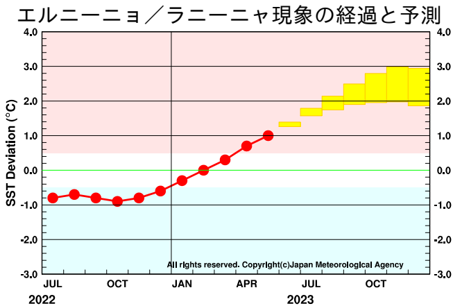
図 1 エルニーニョ監視海域の海面水温の基準値との差の 5 か月移動平均値 5 月までの経過（観測値）を折れ線グラフで、大気海洋結合モデルによる予測結果（70%の確率で入ると予想される範囲）をボックスで示している。指数が赤／青の範囲に入っている期間がエルニーニョ／ラニーニャ現象の発生期間である。エルニーニョ監視海域の海面水温の基準値はその年の前年までの 30 年間の各月の平均値。
