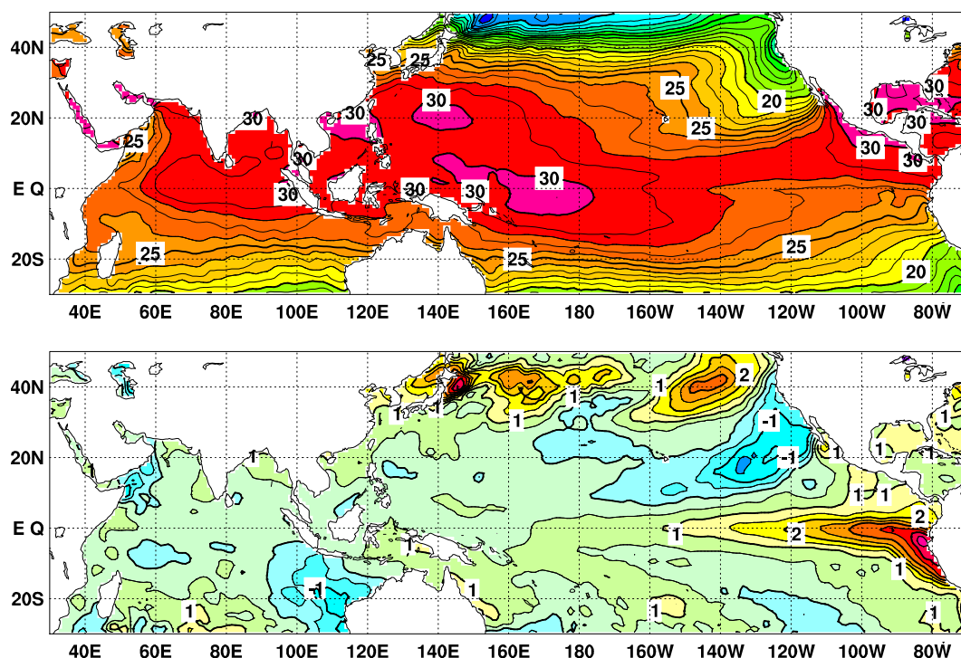
図4 2023年7月の海面水温図（上）及び平年偏差図（下）
