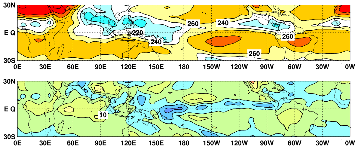
図 9 外向き長波放射量 (OLR) (上) 及び年平均偏差 (下) の分布図 (2023 年 7 月)
