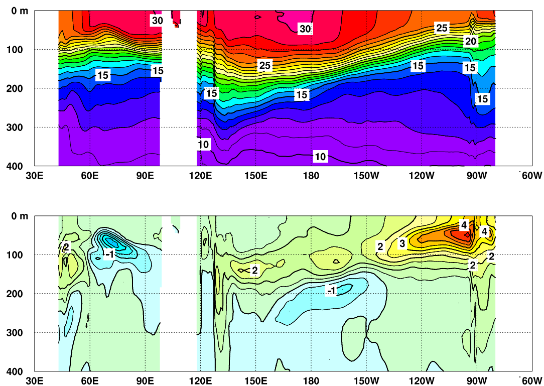
図5 2023年7月のインド洋から太平洋の赤道に沿った水温（上）及び平年偏差（下）の断面図
