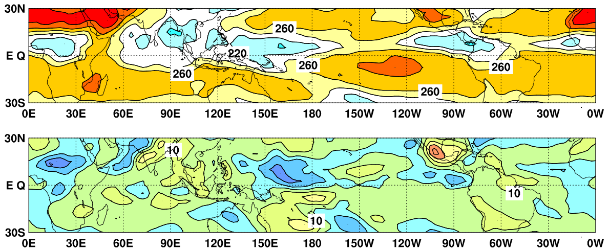
図9 外向き長波放射量 (OLR) (上) 及び平年偏差 (下) の分布図 (2023年6月)
