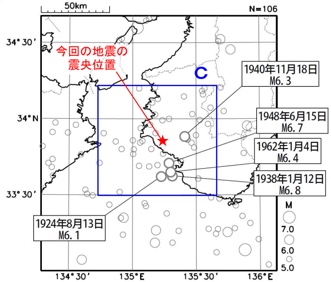
震央分布図 (1919年1月1日～2023年6月30日、 深さ0～100km、M≥5.0)
