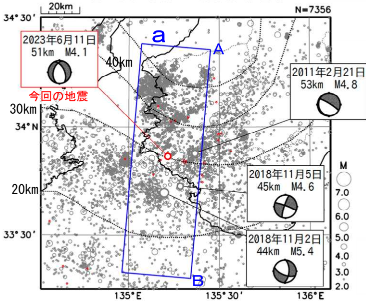
震央分布図 (1997年10月1日～2023年6月30日、 深さ0～80km、M≥2.0) 2023年6月1日以降の地震を赤く表示
